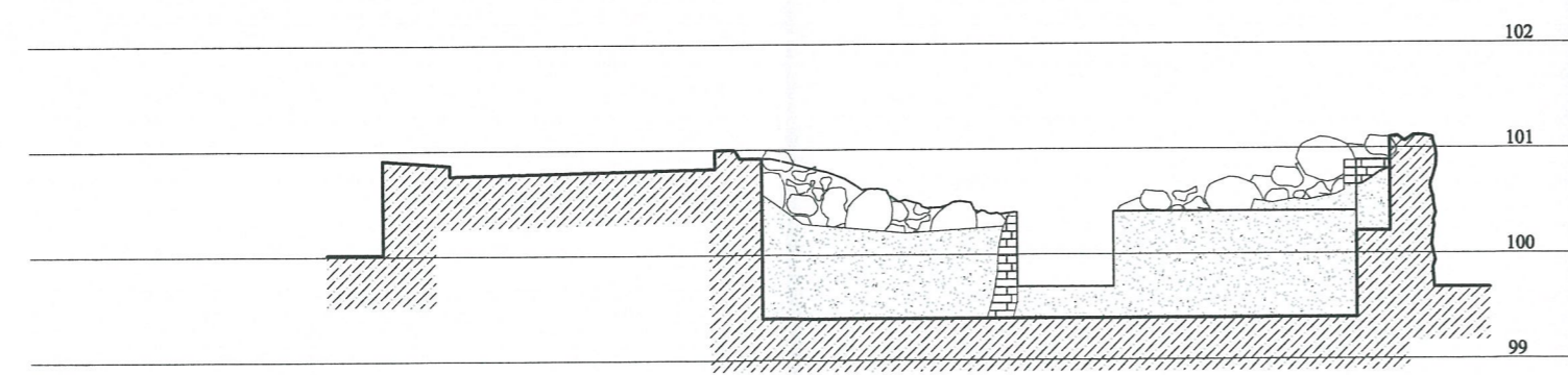
PJŪVIS F-F
