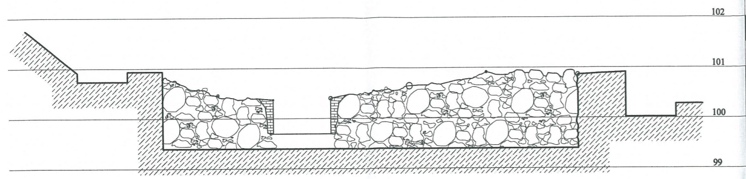
PJŪVIS A-A
