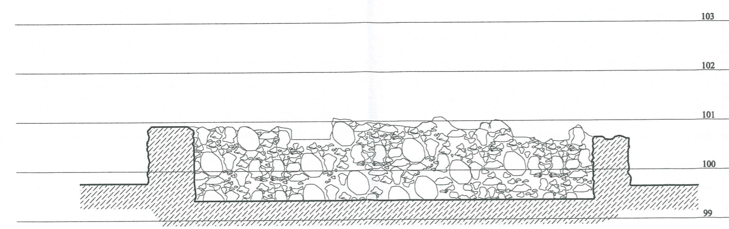
PJŪVIS B-B
