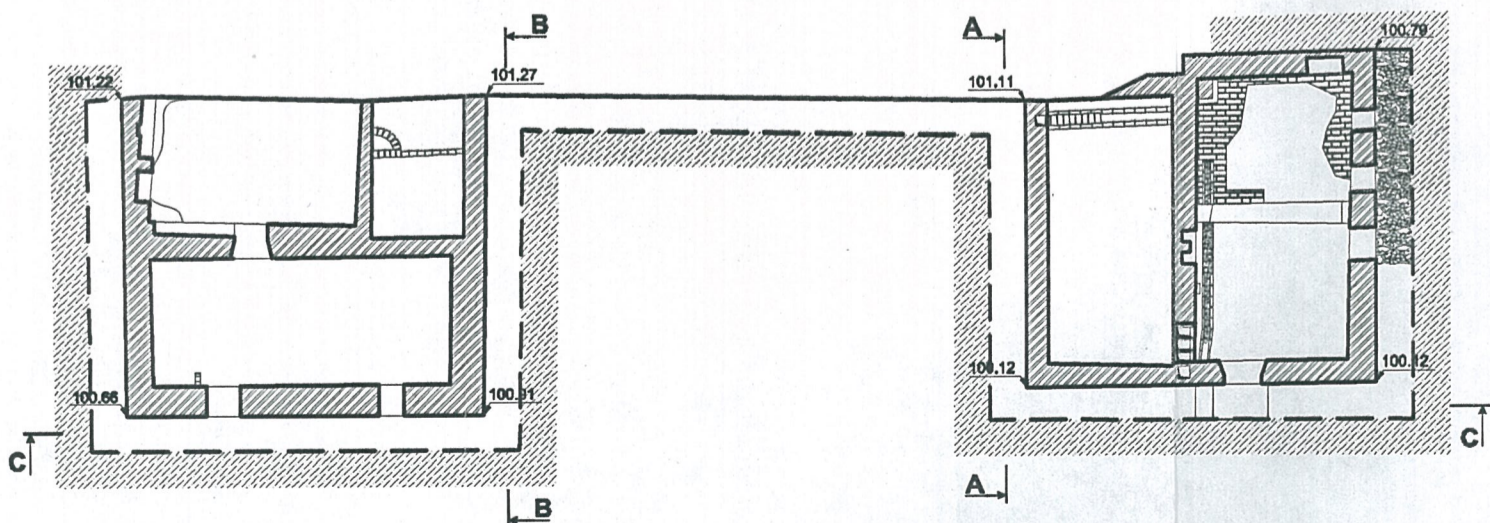
SITUACIJOS PLANAS
