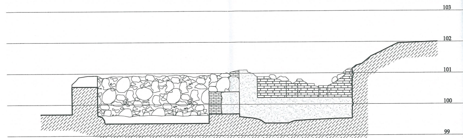
PJŪVIS D-D
