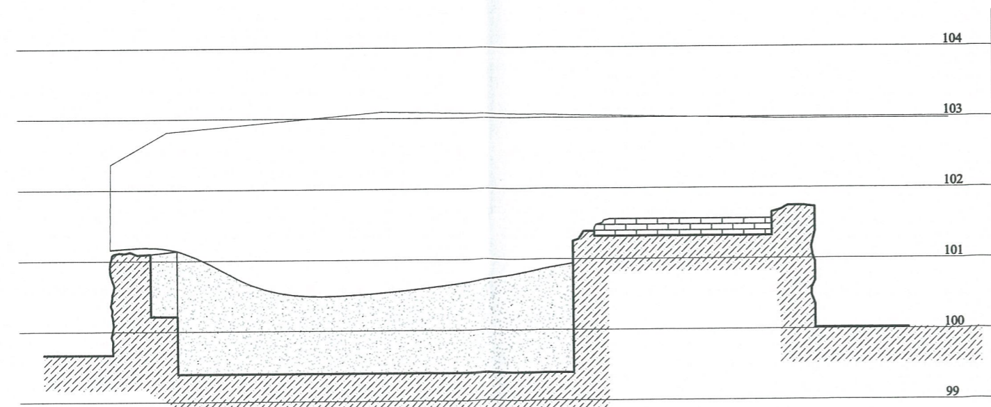
PJŪVIS E-E
