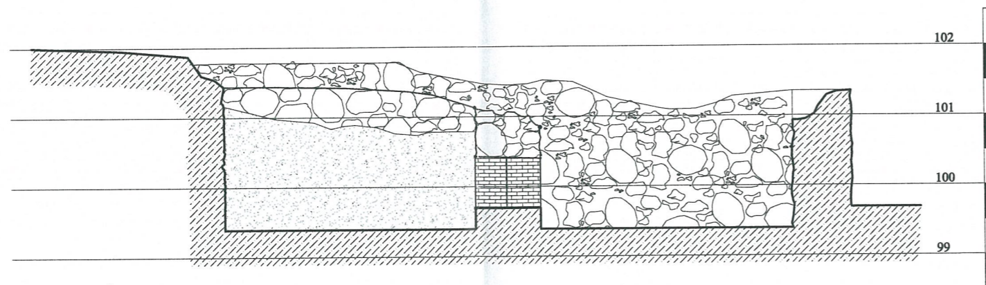
PJŪVIS C-C
