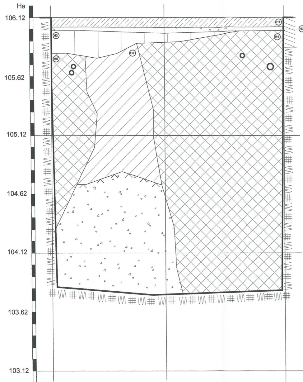
ŠR. 3, P PJŪVIS, M 1:20
