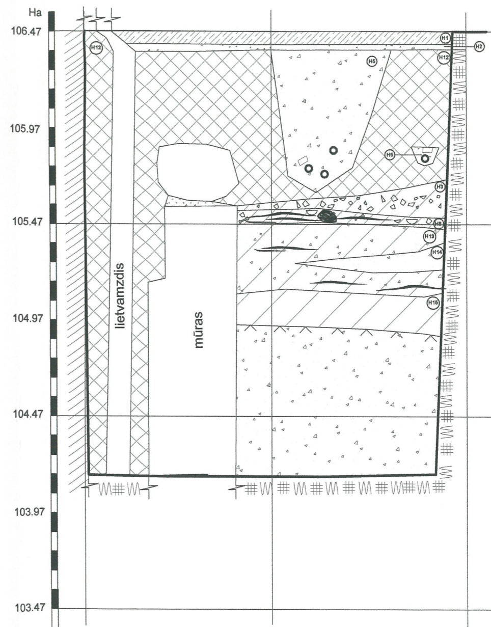
ŠR. 2, P PJŪVIS, M 1:20
