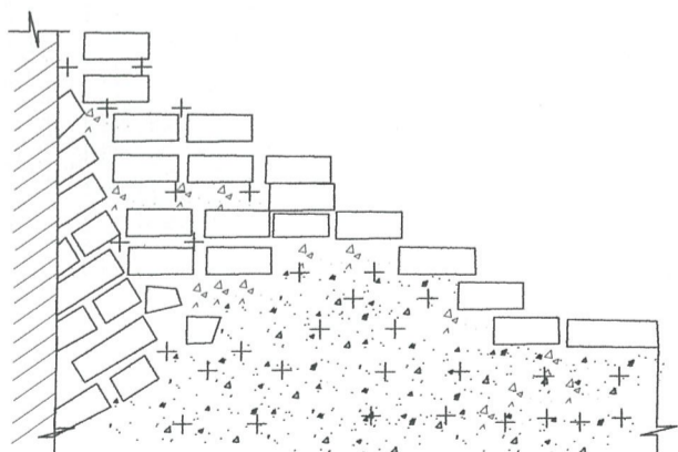
ŠR. 2 prie Š krašto esančio mūro planas iš V pusės, M 1:20
