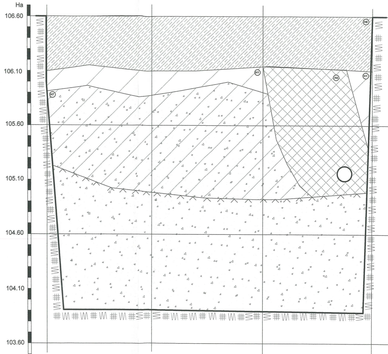
ŠR. 1, P PJŪVIS, M 1:20
