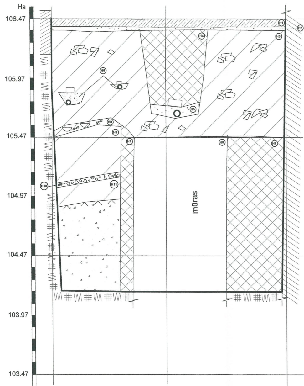
ŠR. 2, Š PJŪVIS, M 1:20
