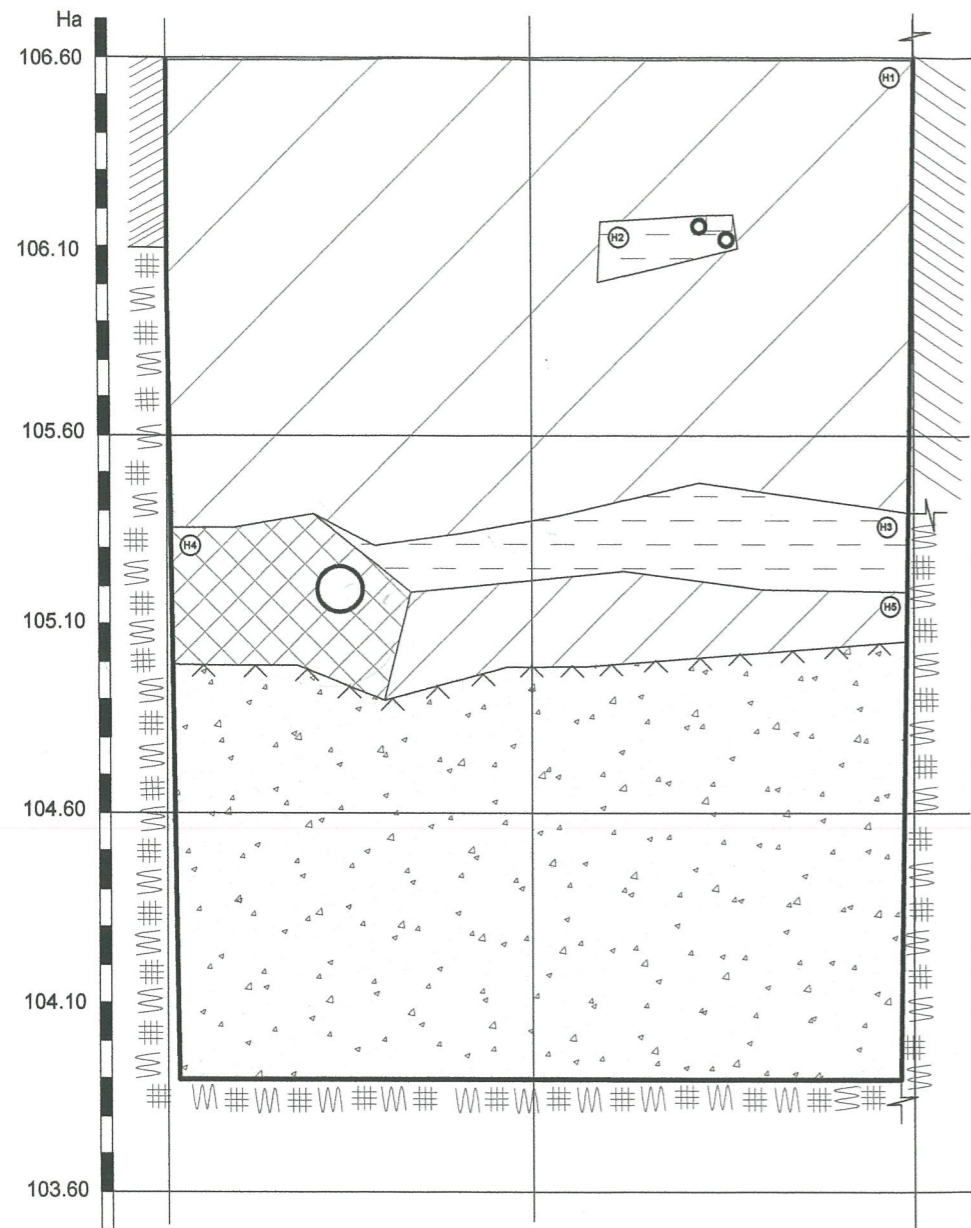
ŠR. 1, V PJŪVIS, M 1:20
