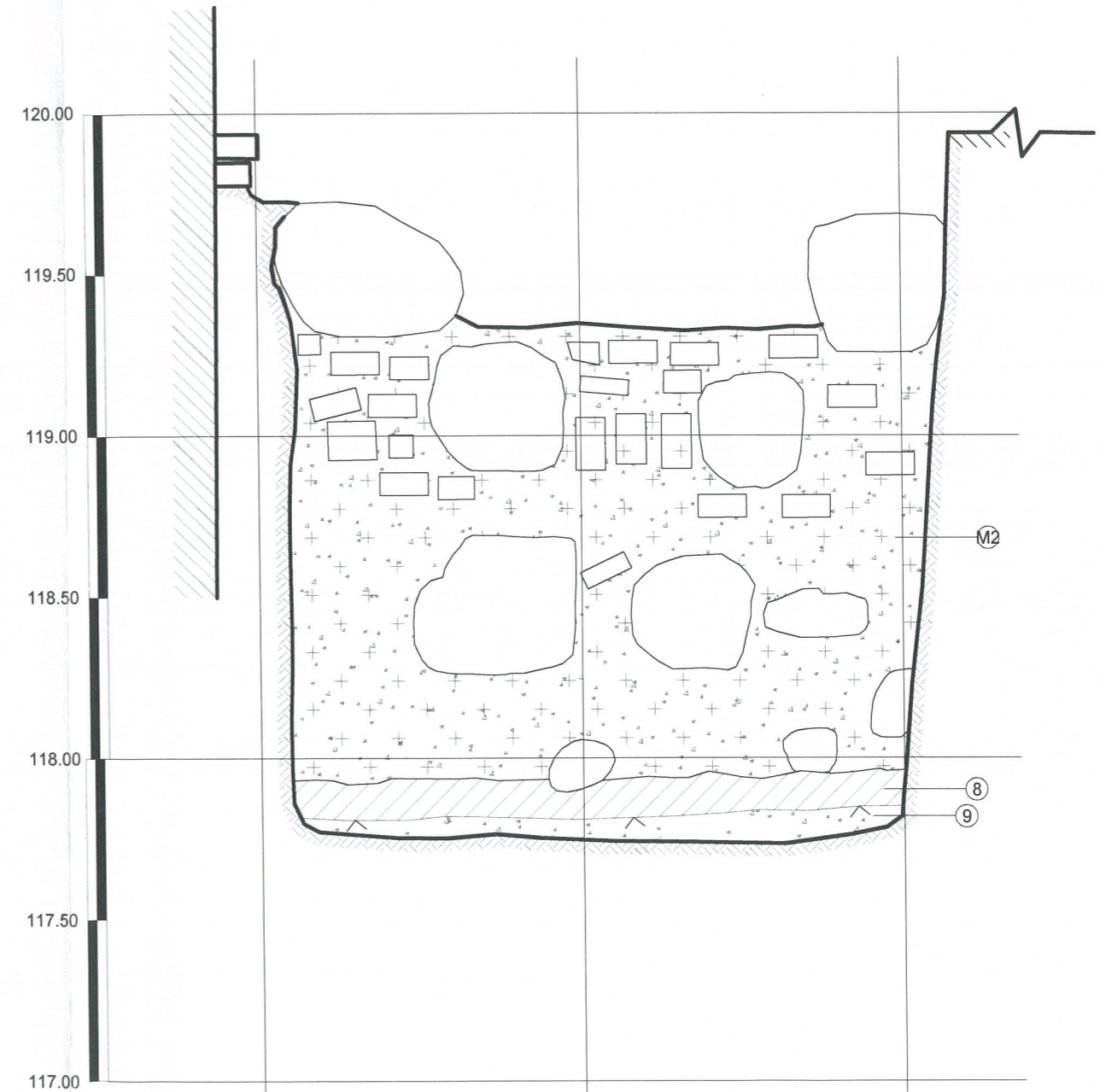
PIETINĖ KRAŠTINĖ PJŪVIS 2-2
