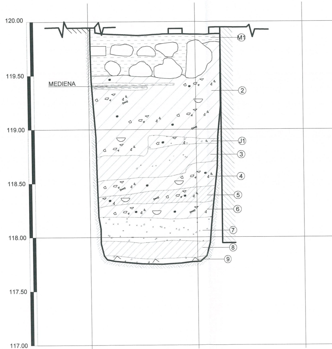
RYTINĖ KRAŠTINĖ PJŪVIS 1-1
