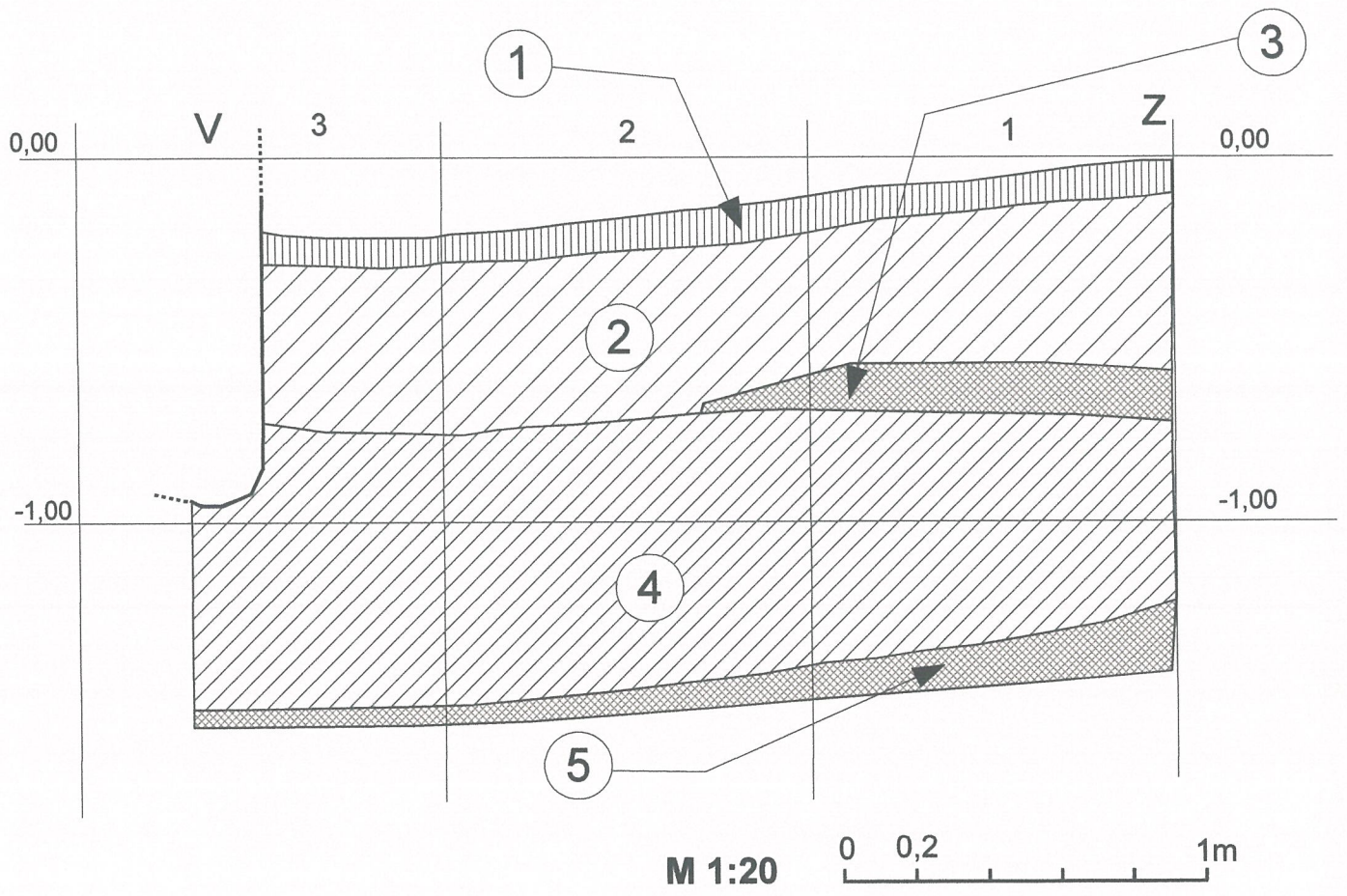
Brėžinys Nr. 20. Archeologiniai tyrinėjimai Šeduvoje, 2010 m. Vytauto g. 19 ir 21. Perkasa Nr. 12. PV sienelės pjūvis.
