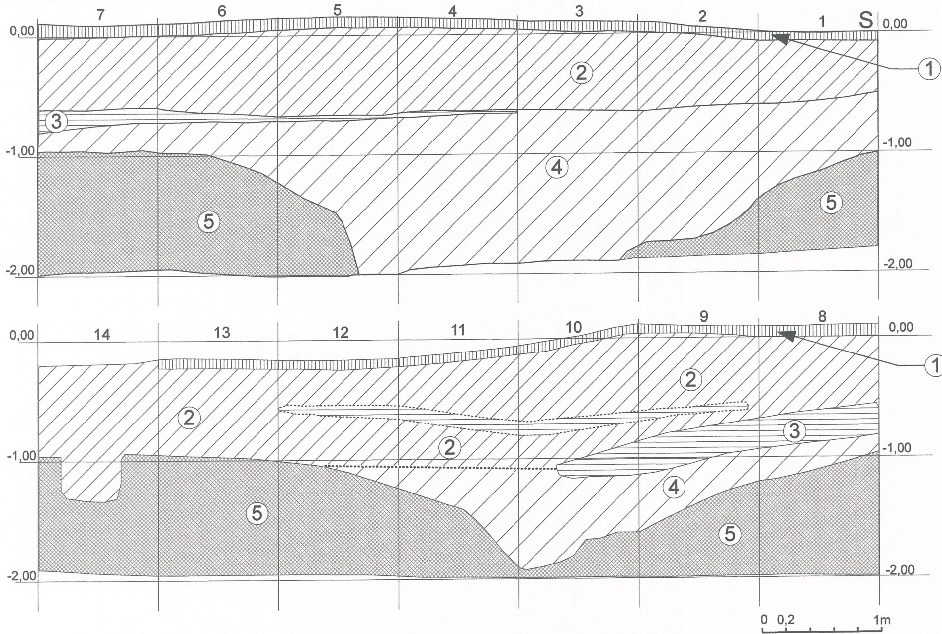
Brėžinys Nr. 15. Archeologiniai tyrinėjimai Šeduvoje, 2010 m. Vytauto g. 17 ir 19A. Perkasa Nr. 9. PV sienelės pjūvis R – S, 1 – 14 m.
