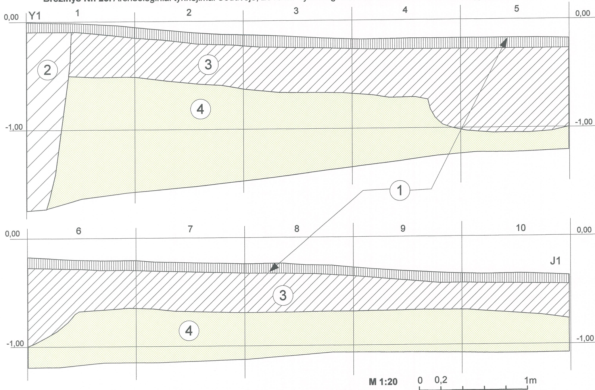
Brėžinys Nr. 25. Archeologiniai tyrinėjimai Šeduvoje, 2010 m. Vytauto g. 33. Perkasa Nr. 18. PV sienelės pjūvis Y1 – J1.
