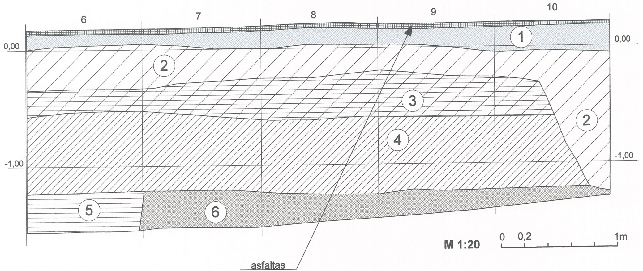
Brėžinys Nr. 12. Archeologiniai tyrinėjimai Šeduvoje, 2010 m. Vytauto g. 8. Perkasa Nr. 7. ŠV sienelės pjūvis M – N, 6 – 10m.
