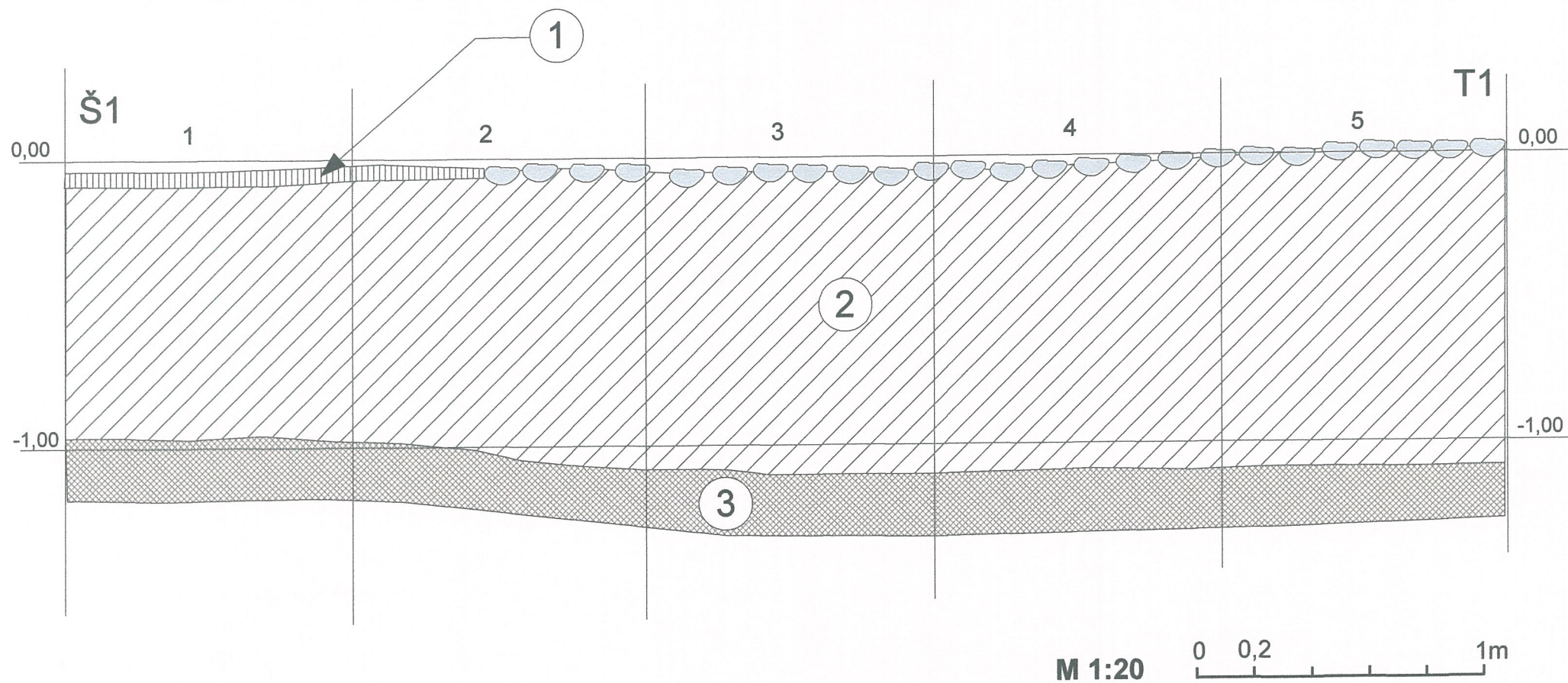
Brėžinys Nr. 33. Archeologiniai tyrinėjimai Šeduvoje, 2010 m. Vilniaus g. 7. Perkasa Nr. 23. P sienelės pjūvis Š1 – T1.
