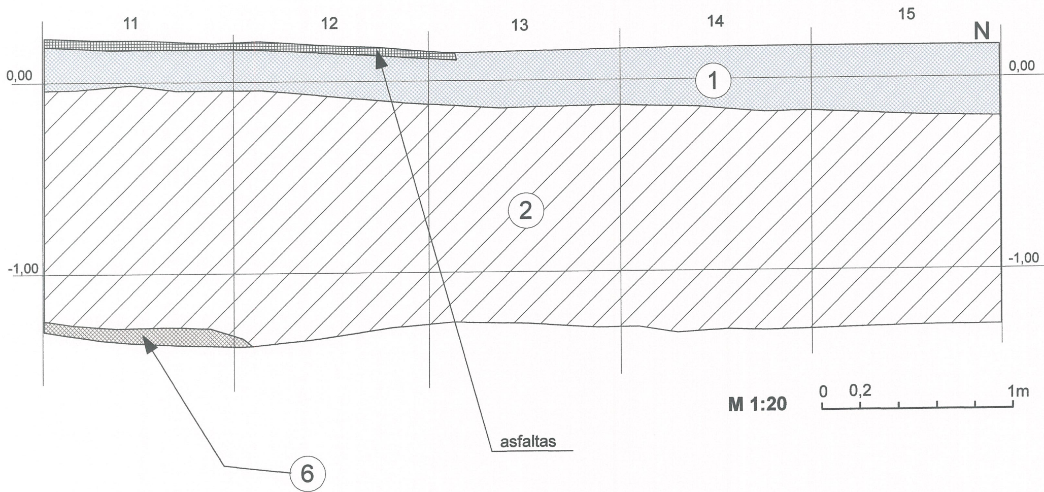
Brėžinys Nr. 13. Archeologiniai tyrinėjimai Šeduvoje, 2010 m. Vytauto g. 8. Perkasa Nr. 7. ŠV sienelės pjūvis M – N, 11 – 15m.
