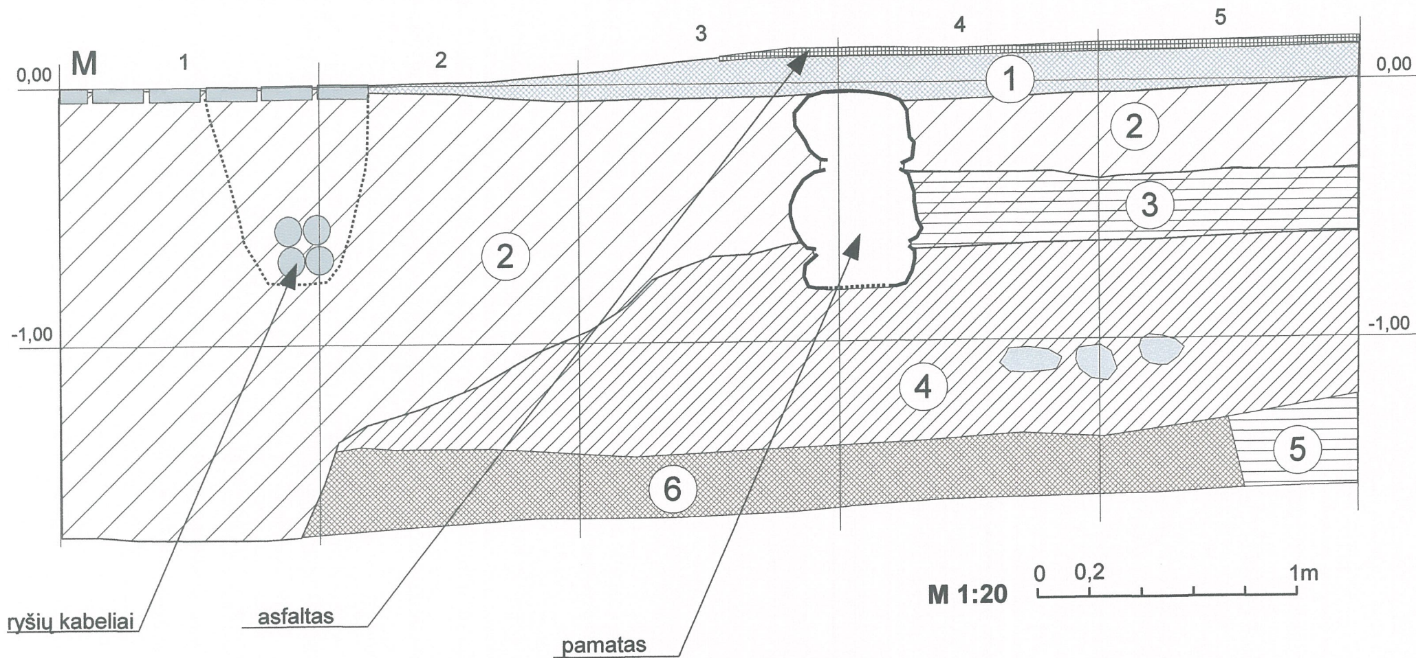
Brėžinys Nr. 11. Archeologiniai tyrinėjimai Šeduvoje, 2010 m. Vytauto g. 8. Perkasa Nr. 7. ŠV sienelės pjūvis M – N, 1 – 5m.
