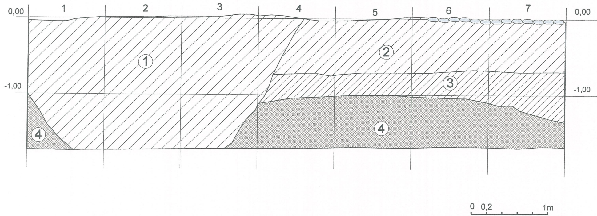
Brėžinys Nr. 35. Archeologiniai tyrinėjimai Šeduvoje, 2010 m. Bažnyčios g. 2 Perkasa Nr. 25. PV sienelės pjūvis V1 – Z1.
