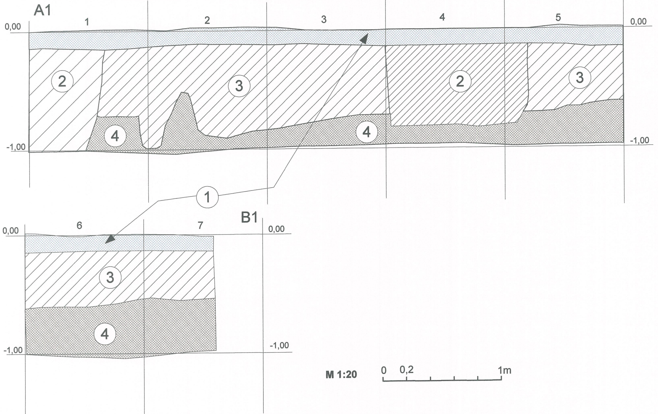
Brėžinys Nr. 21. Archeologiniai tyrinėjimai Šeduvoje, 2010 m. Vytauto g. 22. Perkasa Nr. 13. ŠV sienelės pjūvis A1 – B1.
