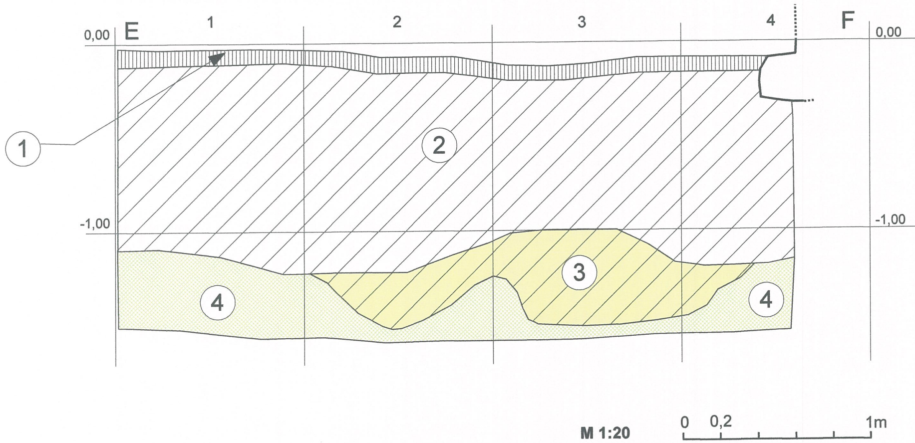
Brėžinys Nr. 8. Archeologiniai tyrinėjimai Šeduvoje, 2010 m. Laisvės a. 25. Perkasa Nr. 3. Š sienelės pjūvis E - F.
