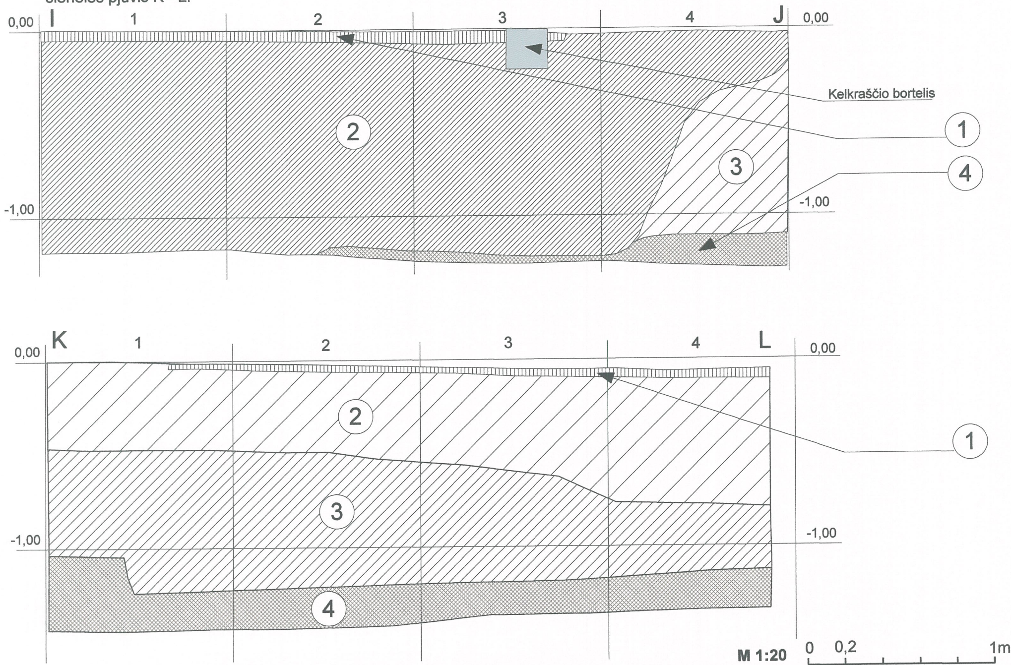
Brėžinys Nr. 10. Archeologiniai tyrinėjimai Šeduvoje, 2010 m. Laisvės a. 26. Perkasos Nr. 5 PR sienelės pjūvis I-J ir perkasos Nr. 6 ŠV sienelės pjūvis K - L.
