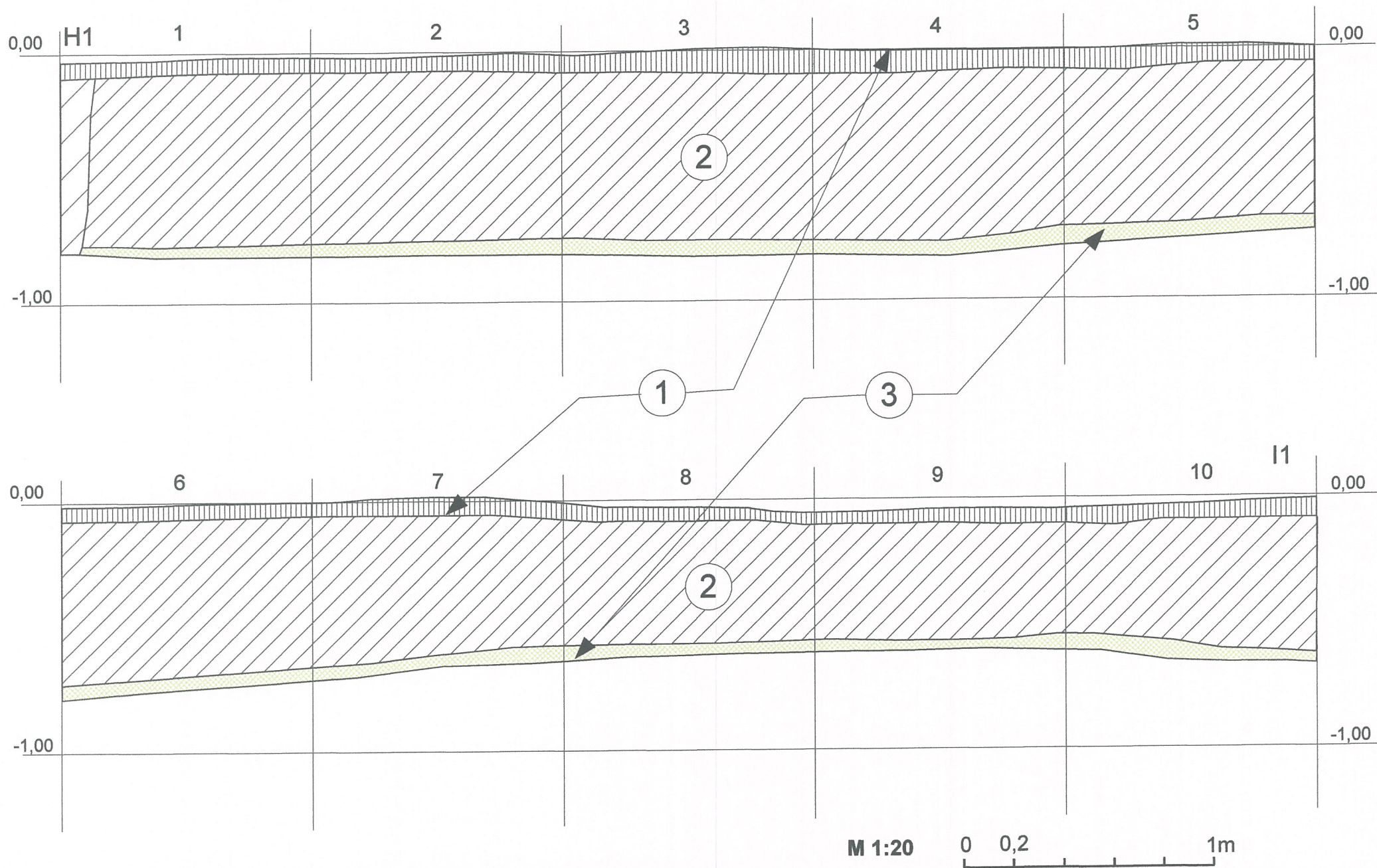
Brėžinys Nr. 24. Archeologiniai tyrinėjimai Šeduvoje, 2010 m. Vytauto g. 31. Perkasa Nr. 17. ŠR sienelės pjūvis H1 – I1.
