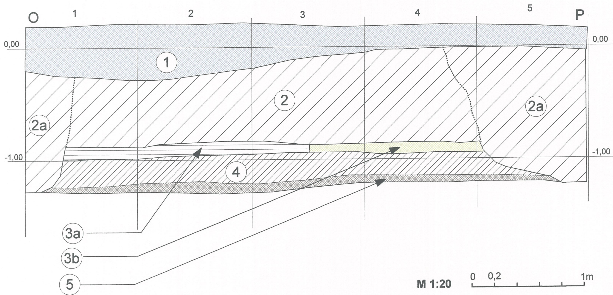
Brėžinys Nr. 14. Archeologiniai tyrinėjimai Šeduvoje, 2010 m. Vytauto g. 8. Perkasa Nr. 8. ŠR sienelės pjūvis O – P.
