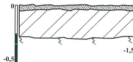
Šūrfas Nr.6 V sienelės pjūvis
