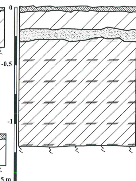
Šūrfas Nr.7 Š sienelės pjūvis
