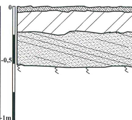
Šūrfas Nr.2 Š sienelės pjūvis
