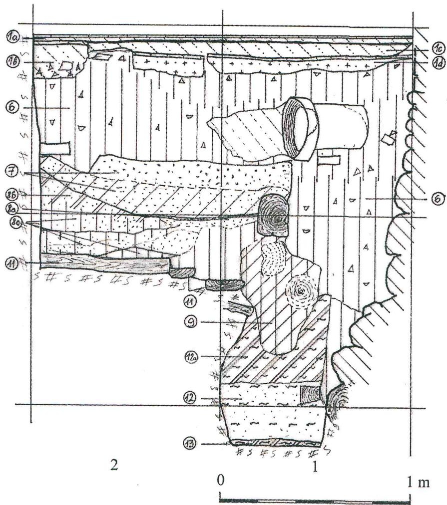
PR sienelēs pjūvis
