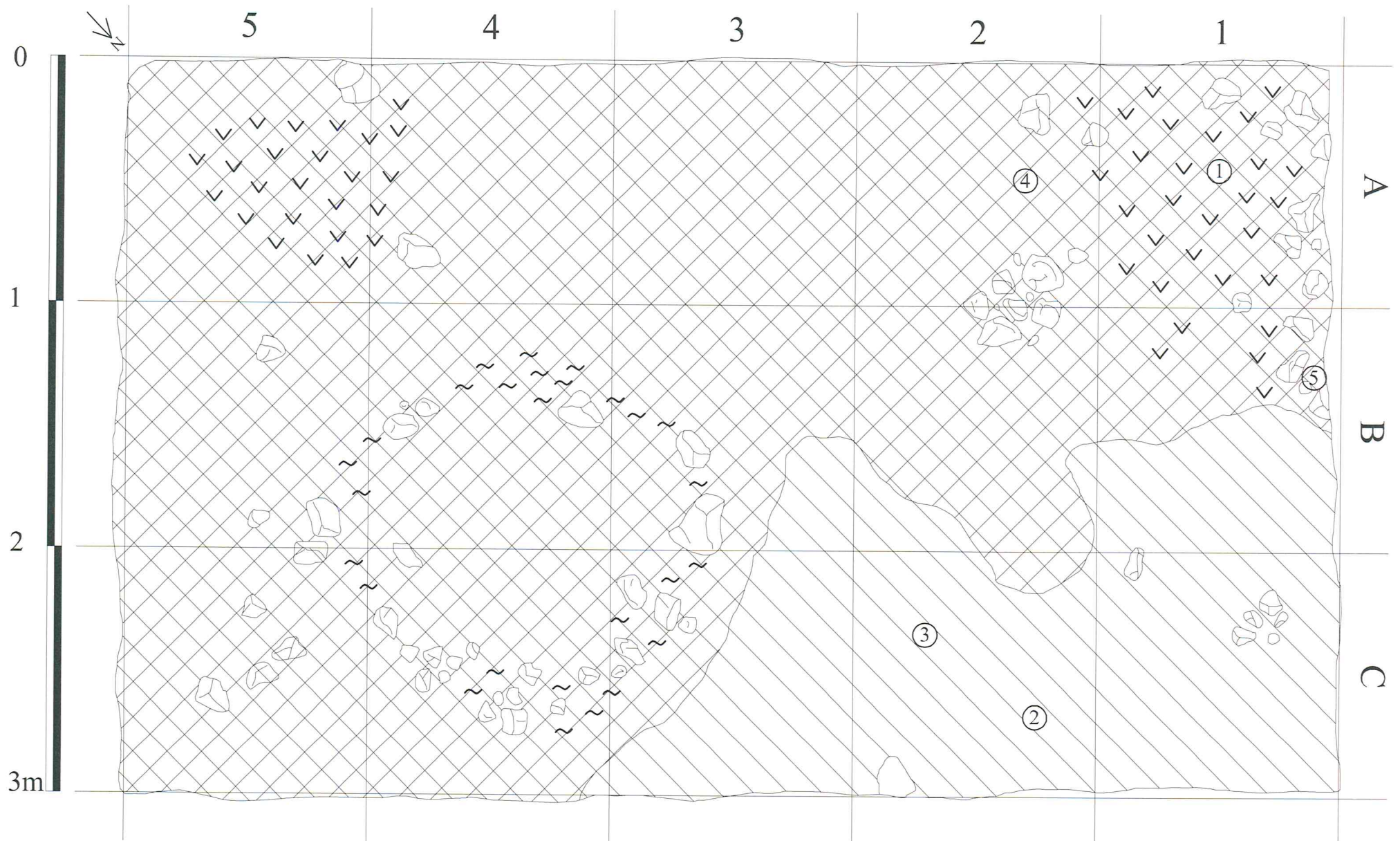
Brėžinys Nr. 1. Ploto Nr. 4 planas, gylis 30 - 40 cm. M 1:20. Braižė D. Balsas
