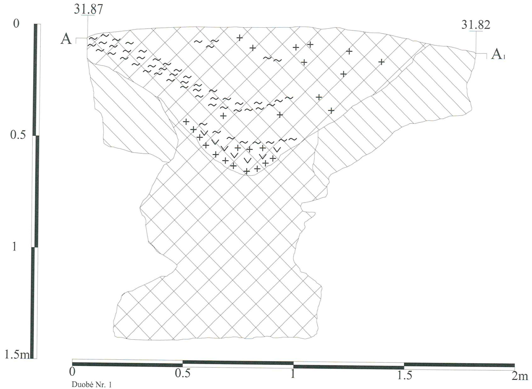
Brėžinys Nr. 8. Duobės Nr. 1 pjūvis A - A 1 . M 1:10. Braižė D. Balsas
