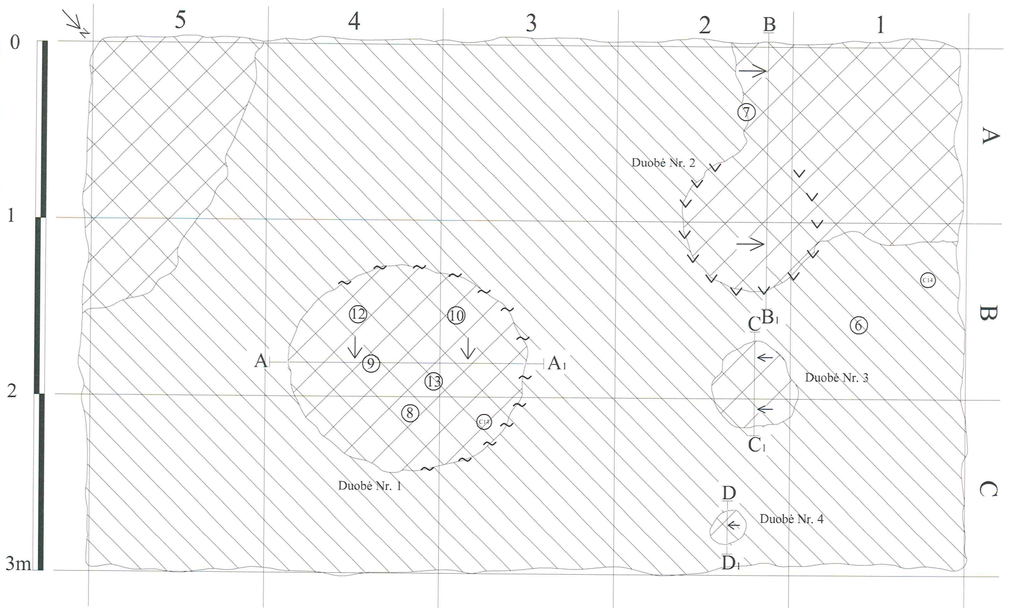
Brėžinys Nr. 2. Ploto Nr. 4 planas, gylis 50 - 55 cm. M 1:20. Braižė D. Balsas
