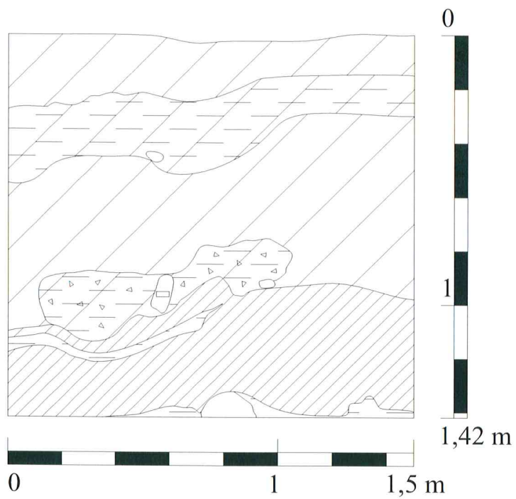
3. Šūrfas Nr. 2, šiaurės rytinēs sienelēs pjūvis. M 1:20
