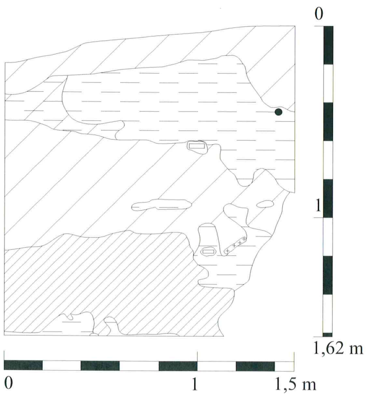
4. Šūrfas Nr. 2, pietrytinēs sienelēs pjūvis. M 1:20
