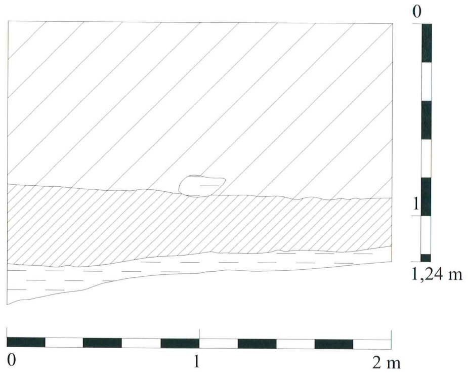
13. Plotas Nr. 6, pietrytinās sienelēs pjūvis. M 1:20
