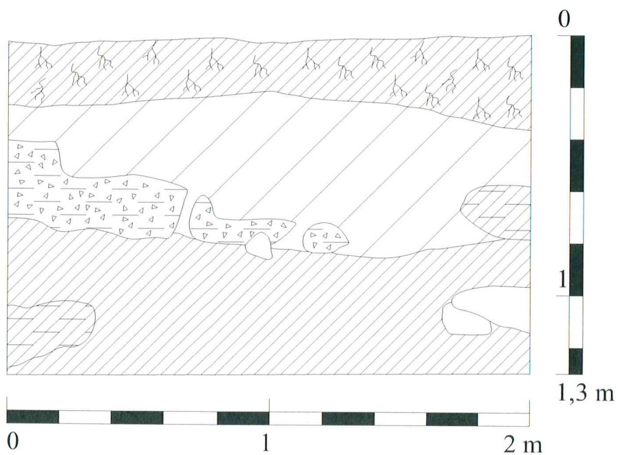
10. Plotas Nr. 3, šiaurės vakarinės sienelės pjūvis ties šiauriniu kampu. M 1:20
