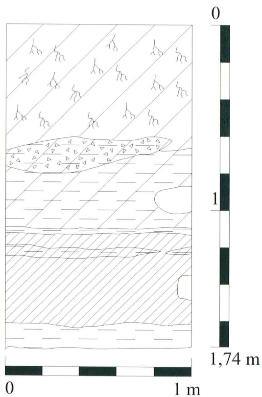
9. Plotas Nr. 3, šiaurės vakarinės sienelės pjūvis ties vakariniu kampu. M 1:20
