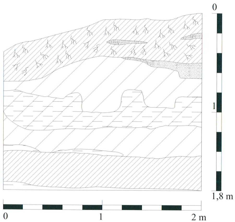
7. Plotas Nr. 1, pietvakarinās sienelēs pjūvis. M 1:20
