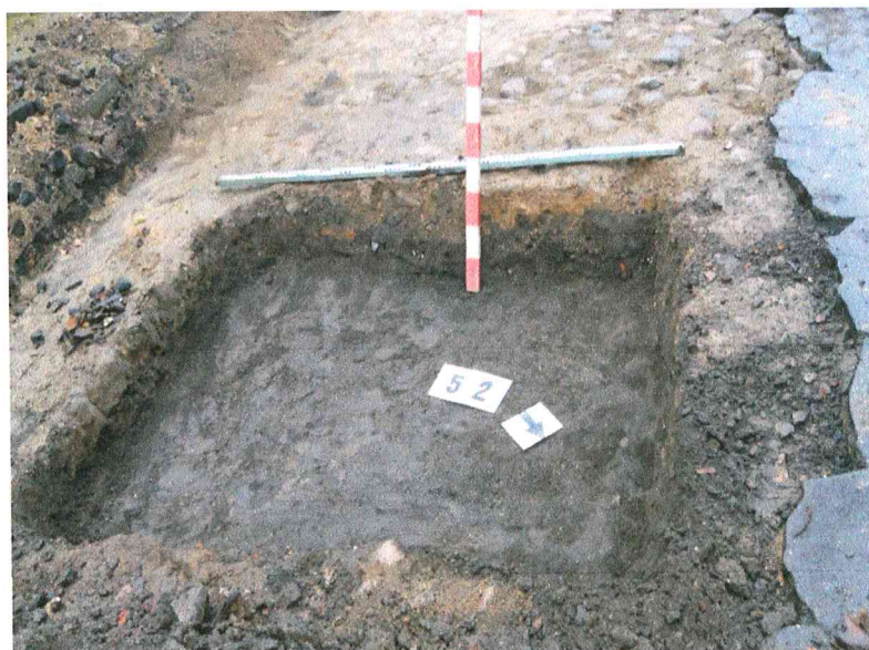
74. Karaimų g. Šurfas Nr.52, iš Š pusės
