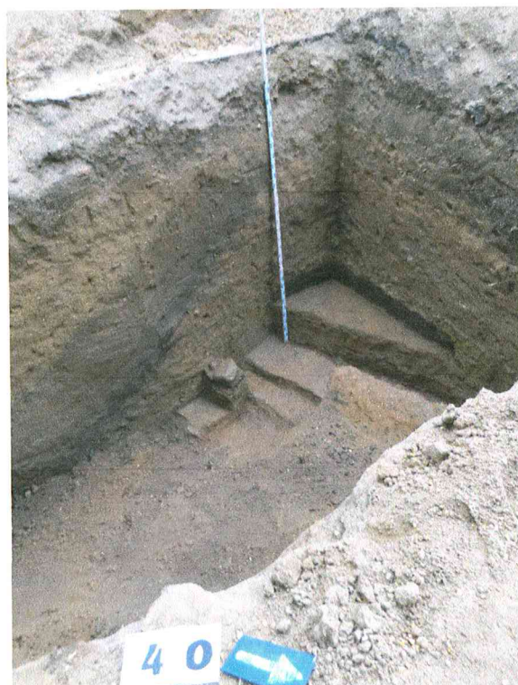
48. Praplatintas šurfas Nr.40, g.3,5 -4,0 m, iš R pusės
