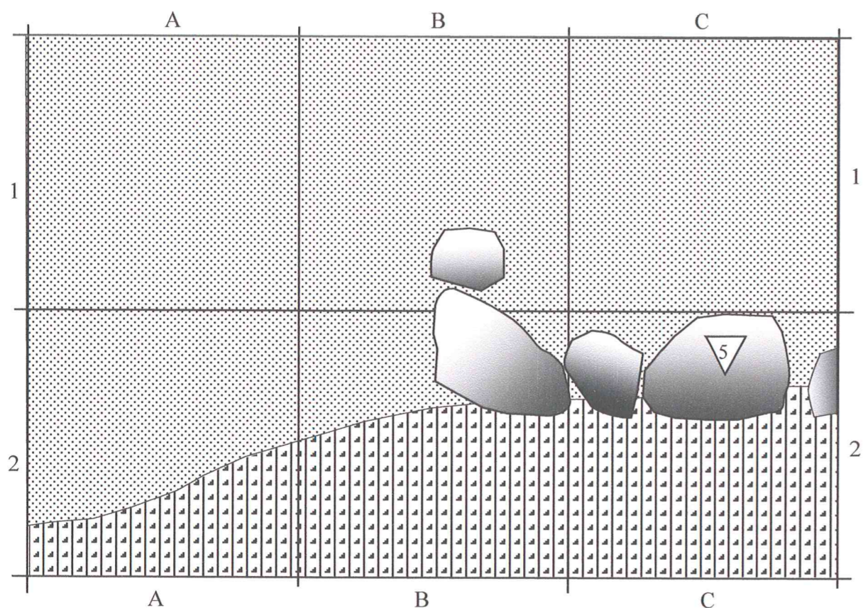
Šūrfas Nr. 10
