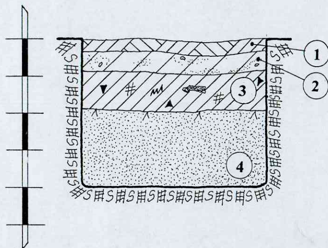
ŠURFAS NR.13. ŠIAURĖS RYTINĖ SIENELĖ. M 1:20
