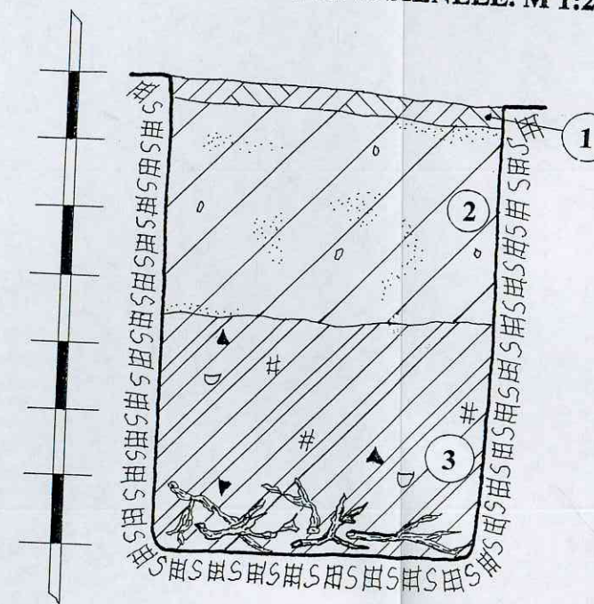
ŠURFAS NR.3. PIETRYTINĖ SIENELĖ. M 1:20
