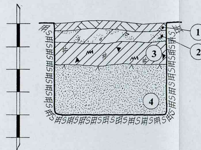
ŠURFAS NR.13. PIETRYTINĖ SIENELĖ. M 1:20
