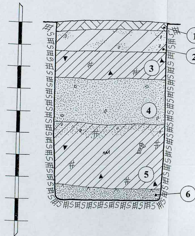
ŠURFAS NR.10. PIETRYTINĖ SIENELĖ. M 1:20
