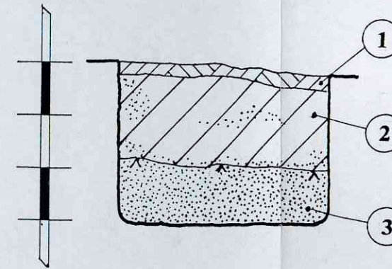
ŠURFAS NR.2. ŠIAURĖS VAKARINĖ SIENELĖ. M 1:20
