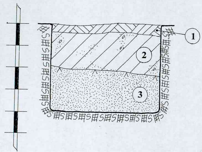
ŠURFAS NR.8. ŠIAURĖS RYTINĖ SIENELĖ. M 1:20
