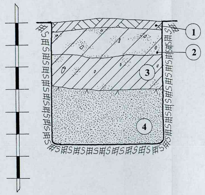
ŠURFAS NR.11. PIETRYTINĖ SIENELĖ. M 1:20
