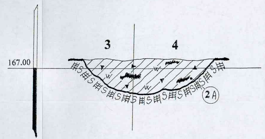
DUOBĖ NR. 9. PJŪVIS D - D. M 1:20
