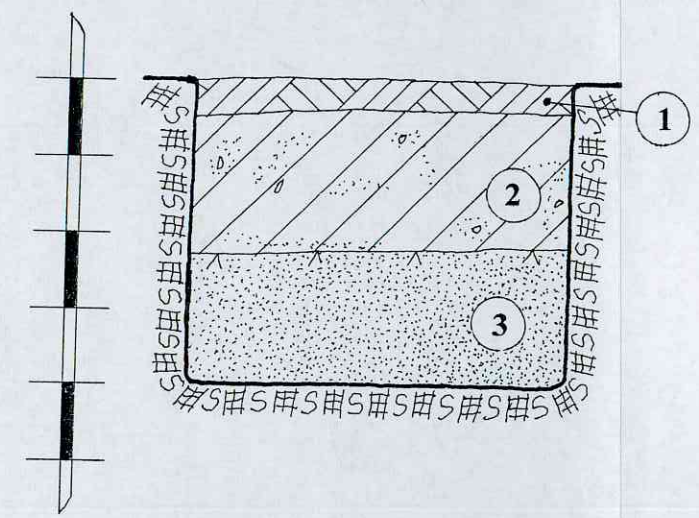
ŠURFAS NR.8. PIETRYTINĖ SIENELĖ. M 1:20
