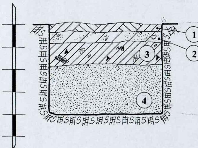
ŠURFAS NR.13. PIETVAKARINĖ SIENELĖ. M 1:20
