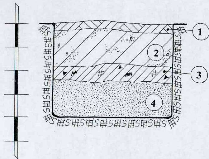
ŠURFAS NR.9. ŠIAURĖS RYTINĖ SIENELĖ. M 1:20
