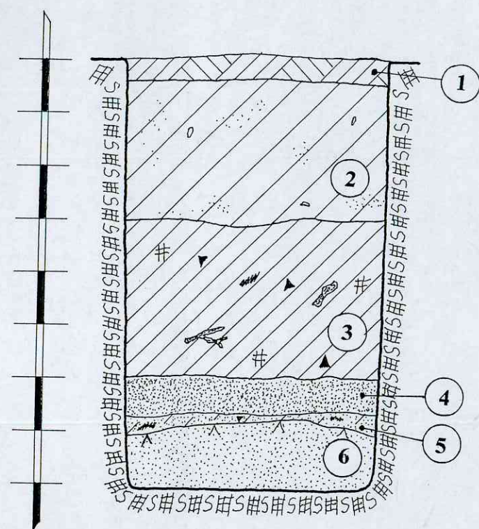
ŠURFAS NR.4. PIETVAKARINĖ SIENELĖ. M 1:20
