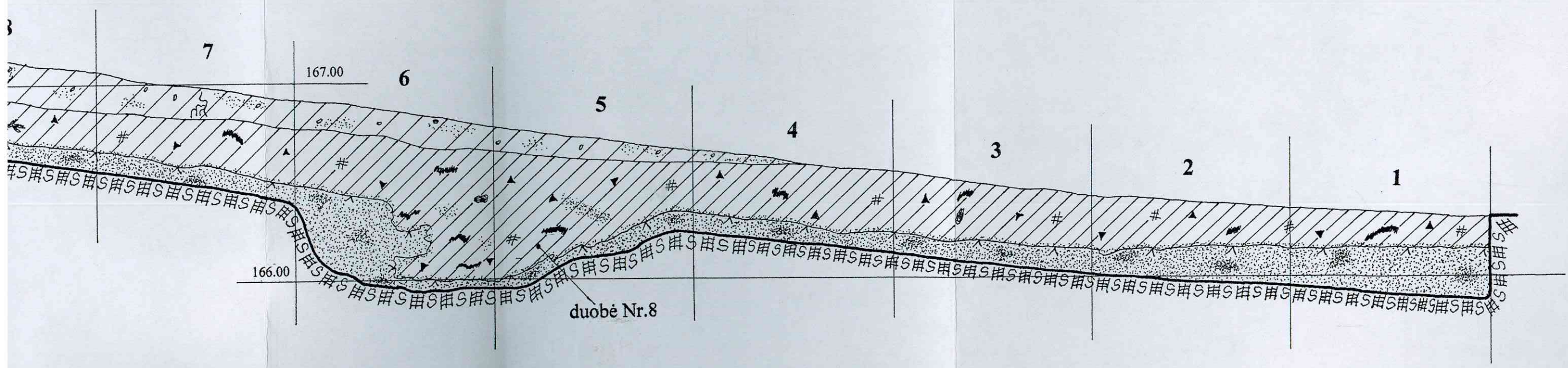
PERKASOS NR.24 PIETRYTINĖ SIENELĖ. M 1:20
