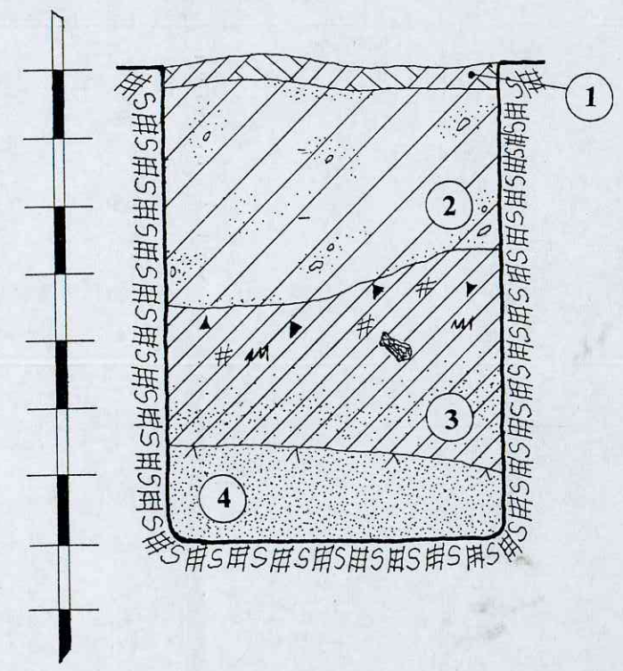
ŠURFAS NR.14. ŠIAURĖS RYTINĖ SIENELĖ. M 1:20
