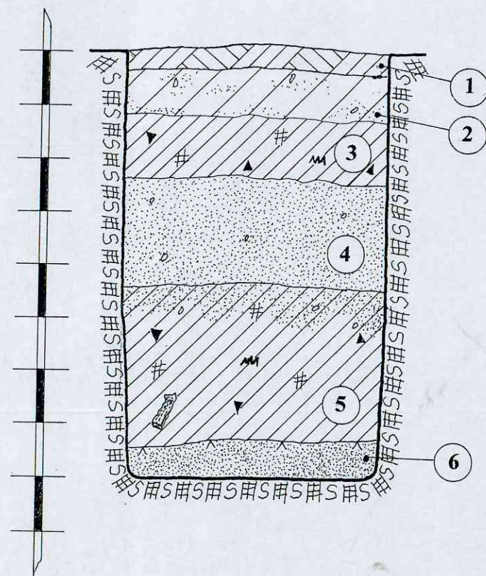
ŠURFAS NR.10. ŠIAURĖS RYTINĖ SIENELĖ. M 1:20
