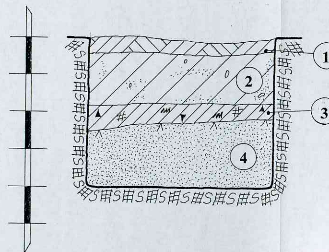
ŠURFAS NR.9. PIETRYTINĖ SIENELĖ. M 1:20
