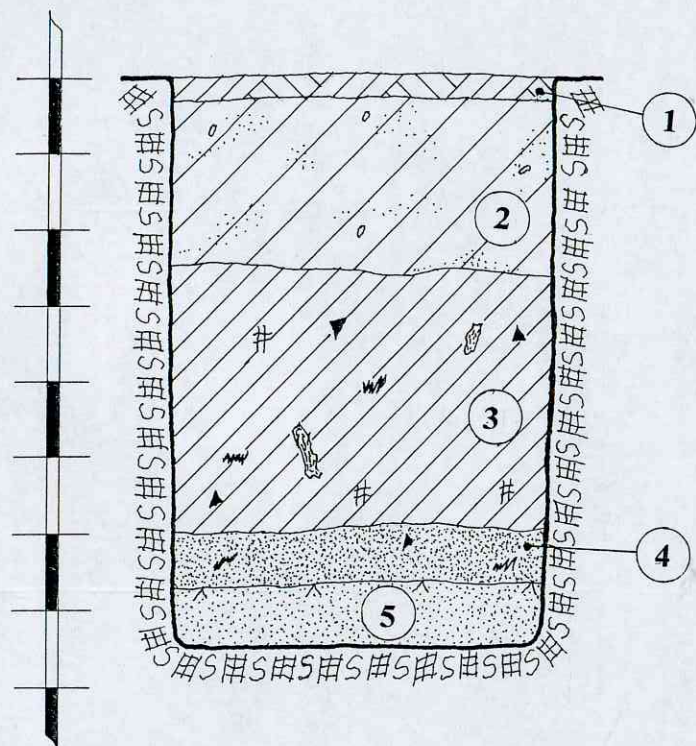
ŠURFAS NR.6. ŠIAURĖS RYTINĖ SIENELĖ. M 1:20
