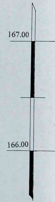
DUOBĖ NR. 8. PJŪVIS C - C. M 1:20
