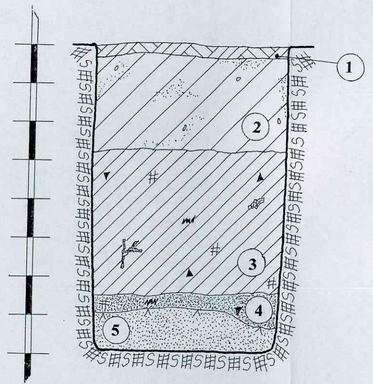
ŠURFAS NR.6. ŠIAURĖS VAKARINĖ SIENELĖ. M 1:20
