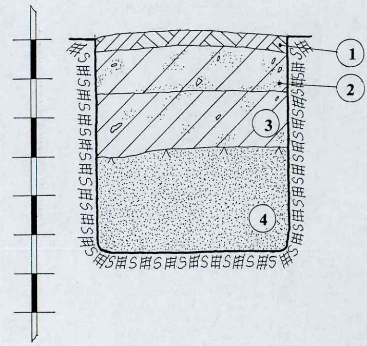
ŠURFAS NR.11. ŠIAURĖS RYTINĖ SIENELĖ. M 1:20
