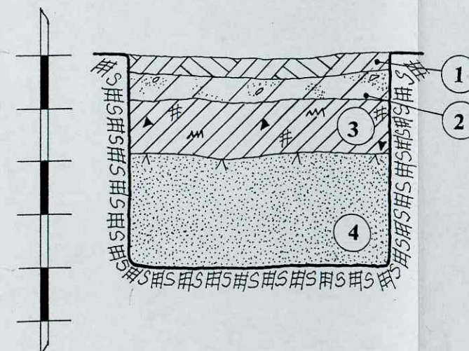
ŠURFAS NR.13. ŠIAURĖS VAKARINĖ SIENELĖ. M 1:20
