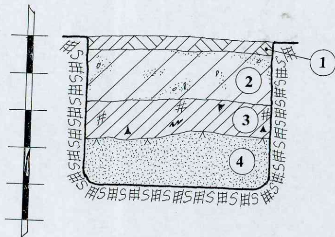
ŠURFAS NR.7. PIETVAKARINĖ SIENELĖ. M 1:20
