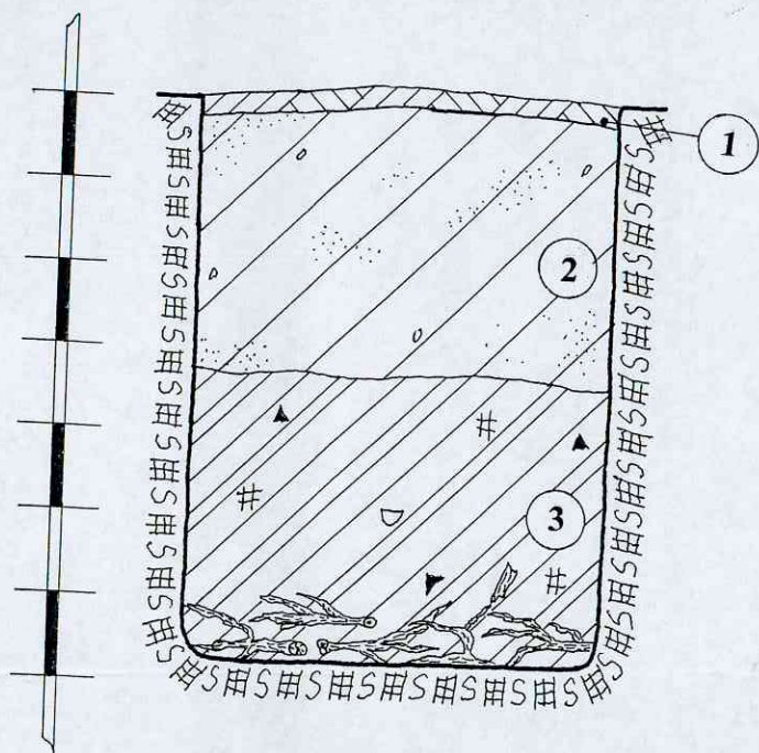
ŠURFAS NR.3. PIETVAKARINĖ SIENELĖ. M 1:20
