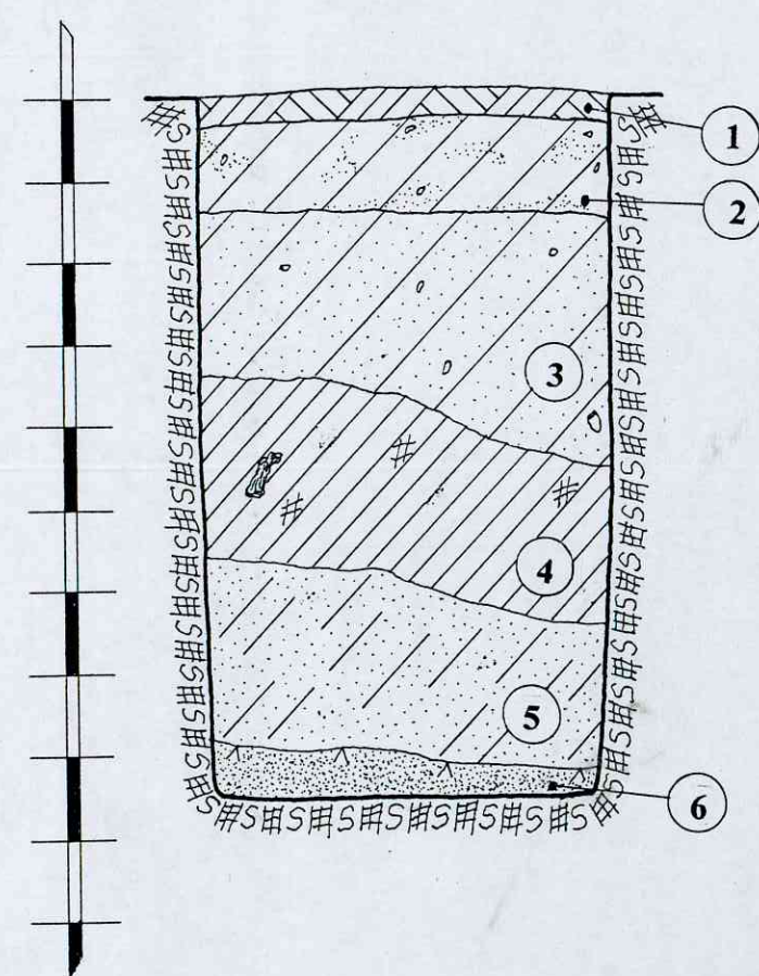
ŠURFAS NR.12. ŠIAURĖS RYTINĖ SIENELĖ. M 1:20
