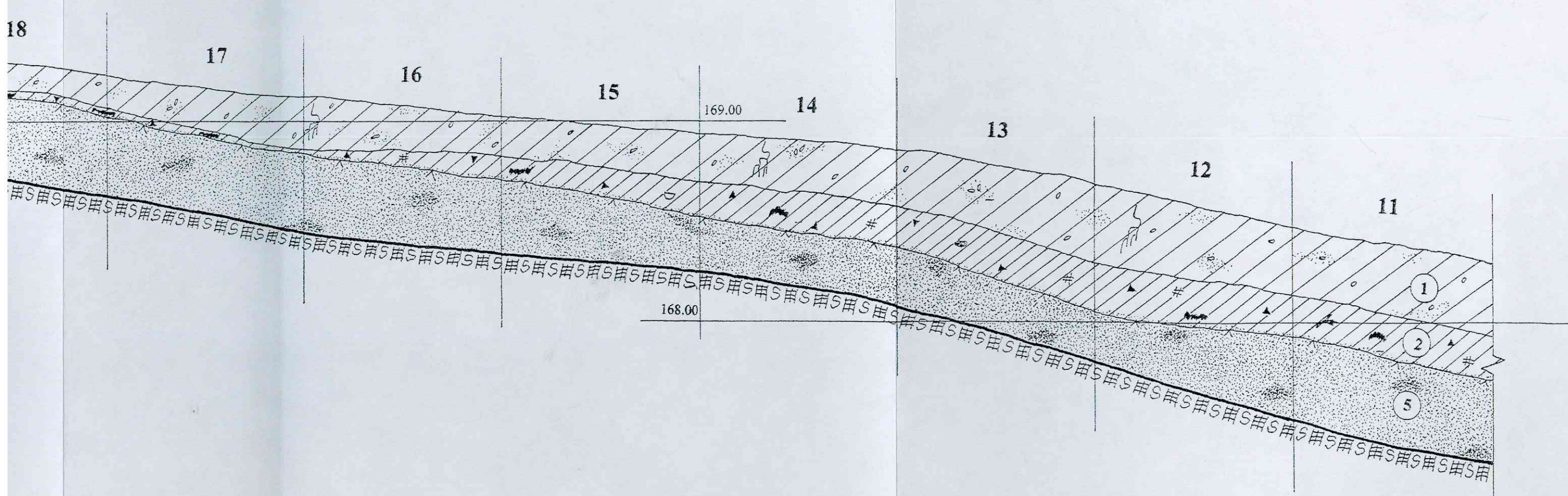
PERKASOS NR.28 PIETRYTINĖ SIENELĖ, METRAI 11-20. M 1:20
