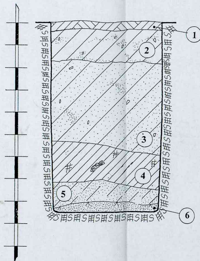
ŠURFAS NR.12. PIETVAKARINĖ SIENELĖ. M 1:20
