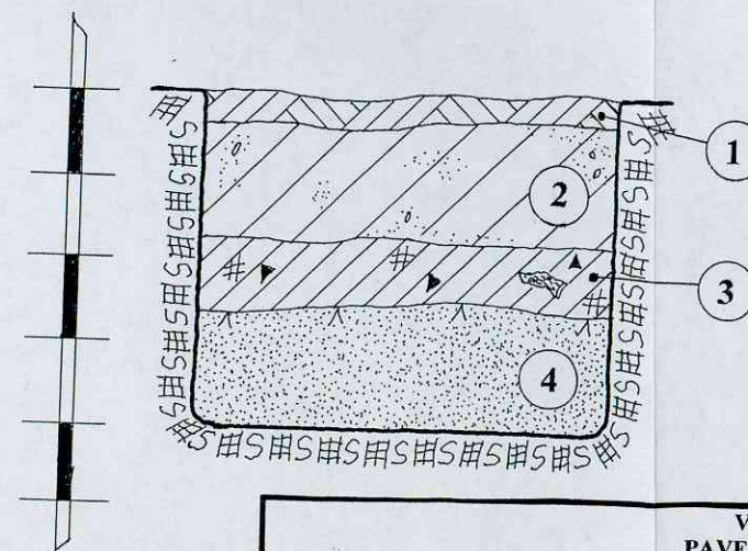
ŠURFAS NR.7. ŠIAURĖS VAKARINĖ SIENELĖ. M 1:20
