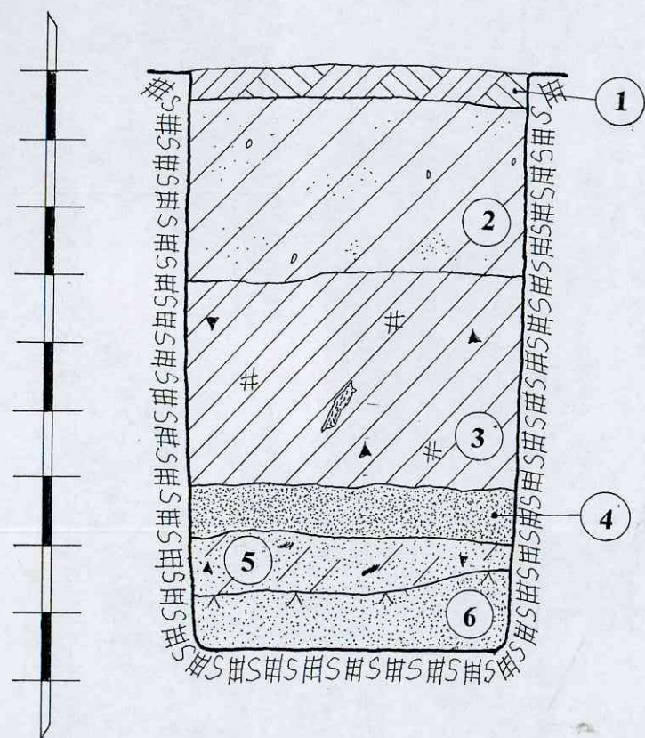
ŠURFAS NR.4. ŠIAURĖS RYTINĖ SIENELĖ. M 1:20
