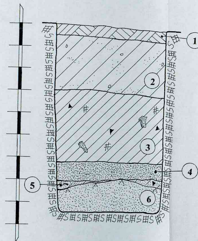
ŠURFAS NR.4. PIETRYTINĖ SIENELĖ. M 1:20
