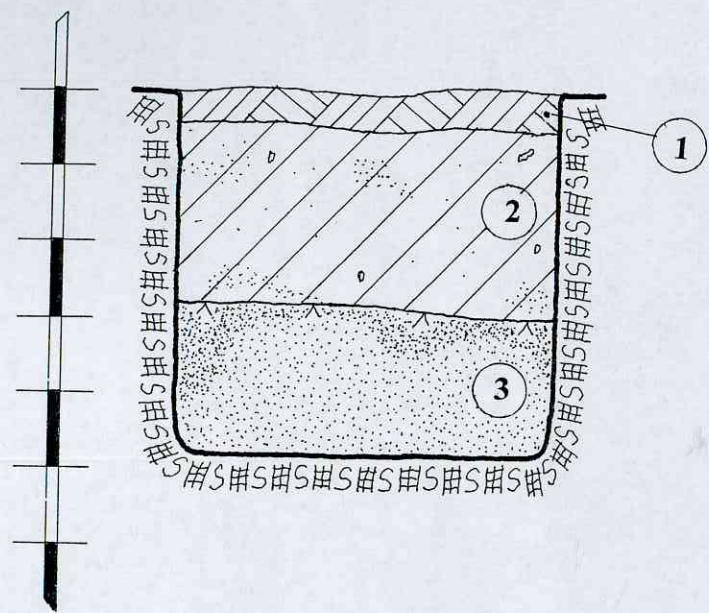
ŠURFAS NR.5. ŠIAURĖS RYTINĖ SIENELĖ. M 1:20
