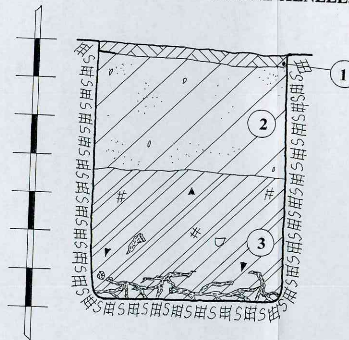
ŠURFAS NR.3. ŠIAURĖS VAKARINĖ SIENELĖ. M 1:20
