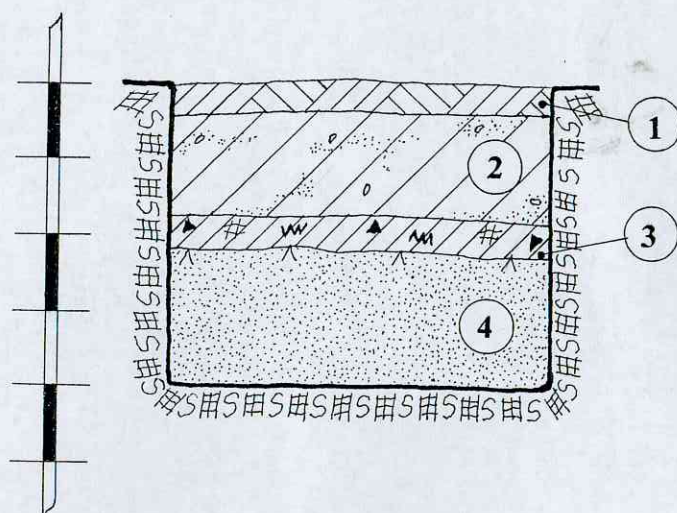
ŠURFAS NR.9. PIETVAKARINĖ SIENELĖ. M 1:20
