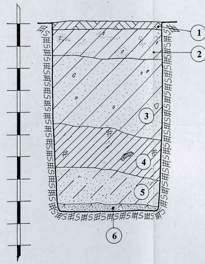
ŠURFAS NR.12. PIETRYTINĖ SIENELĖ. M 1:20
