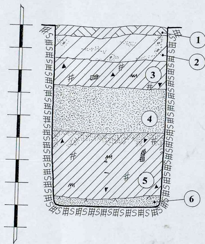
ŠURFAS NR.10. PIETVAKARINĖ SIENELĖ. M 1:20
