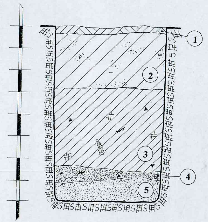
ŠURFAS NR.6. PIETVAKARINĖ SIENELĖ. M 1:20
