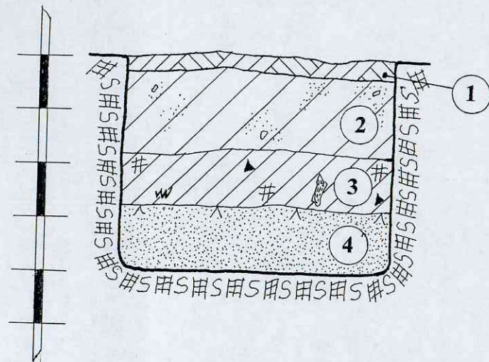
ŠURFAS NR.7. ŠIAURĖS RYTINĖ SIENELĖ. M 1:20
