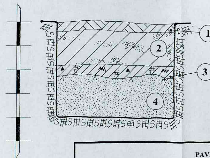
ŠURFAS NR.9. ŠIAURĖS VAKARINĖ SIENELĖ. M 1:20
