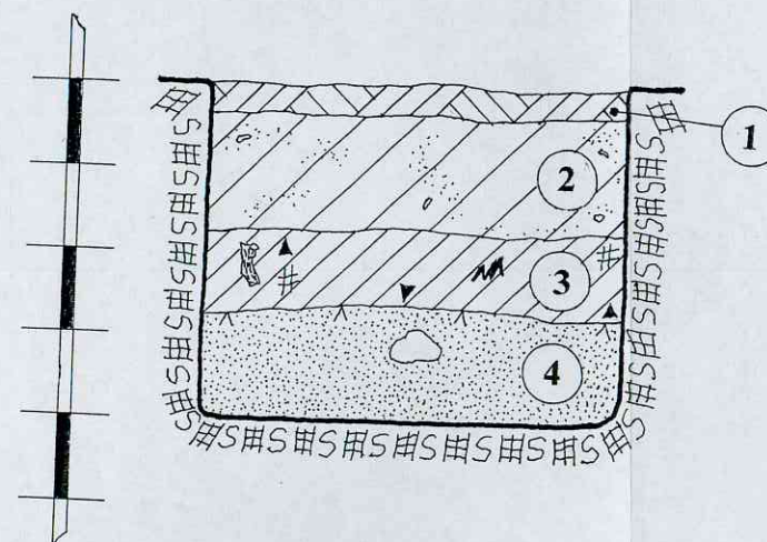
ŠURFAS NR.7. PIETRYTINĖ SIENELĖ. M 1:20
