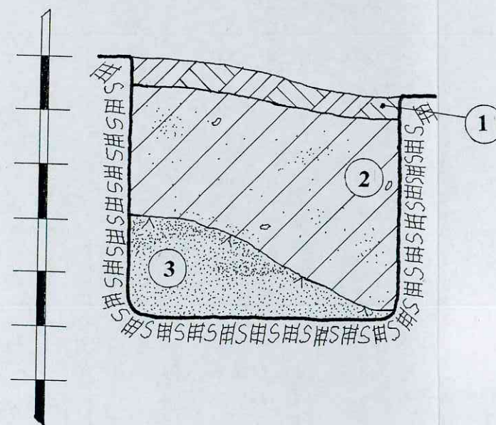
ŠURFAS NR.5. PIETRYTINĖ SIENELĖ. M 1:20
