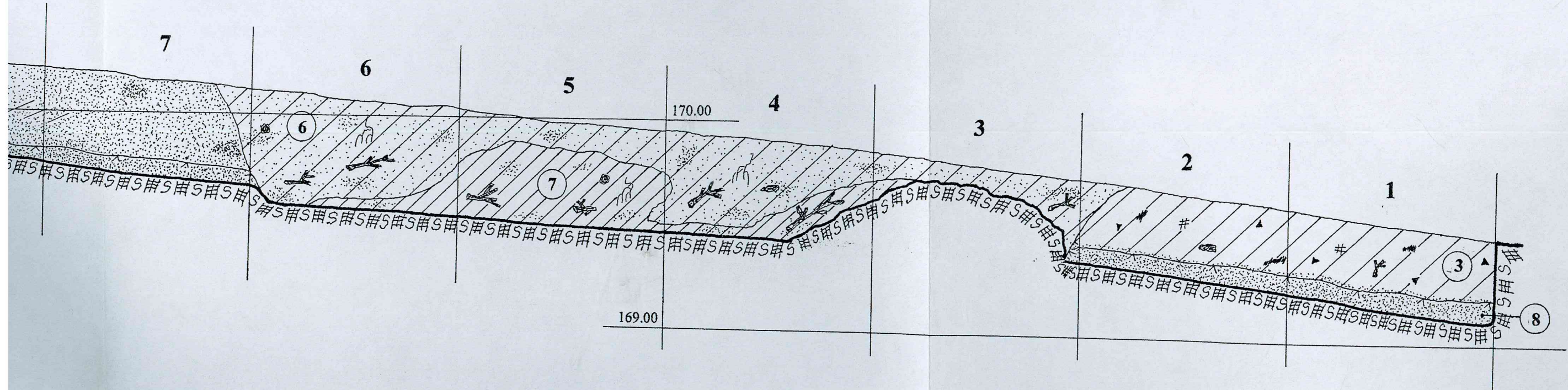
PERKASOS NR.19 PIETRYTINĖ SIENELĖ. M 1:20
