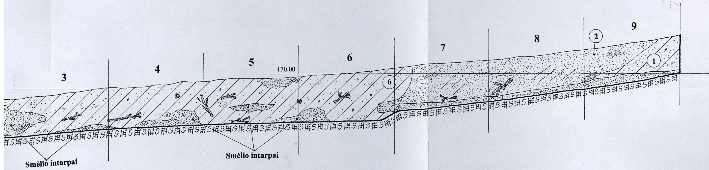
PERKASOS NR.19 ŠIAURĖS VAKARINĖ SIENELĖ. M 1:20
