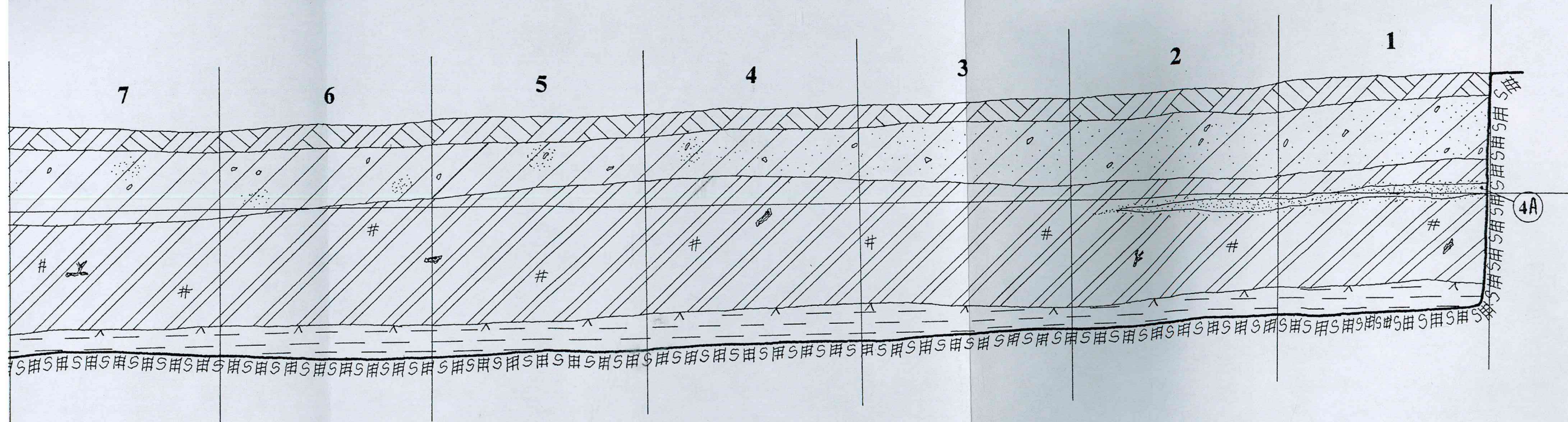
PIETVAKARINĖ SIENELĖ. M 1:20
