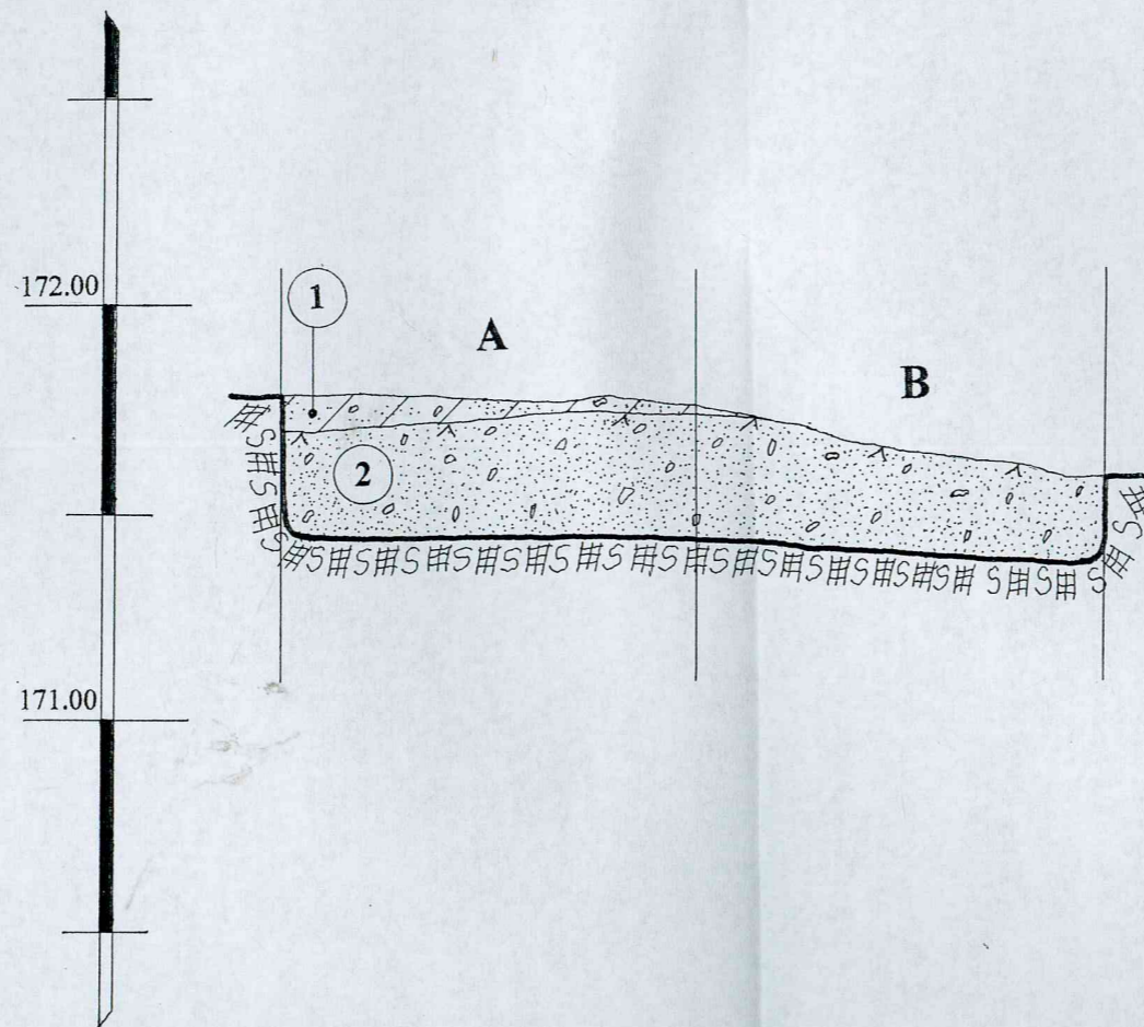
PERKASOS Nr.4 ŠIAURĖS VAKARINĖ SIENELĖ. M 1:20
