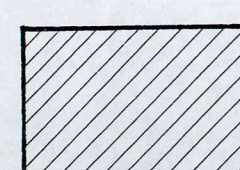
JUODA ŽEMĖ
