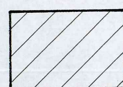
PILKA ŽEMĖ
