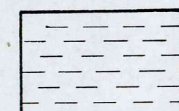
MOLIS
