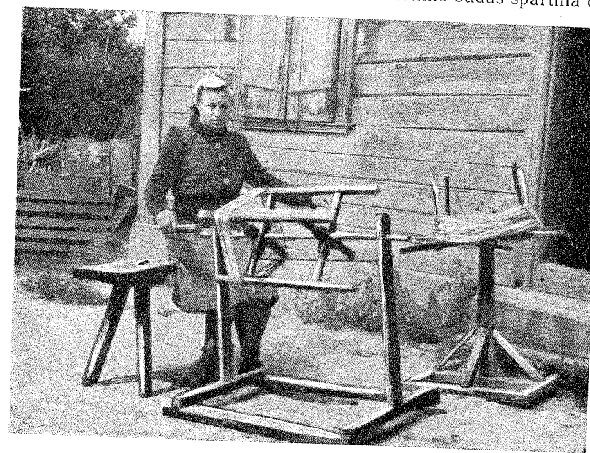
19 pav. Vytuvai (vytuškos) ir krijelis
