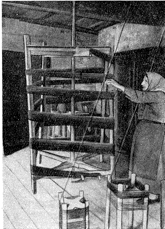
23 pav. Kilnojamieji mestuvai Pandėlio raj., Taručių k.
