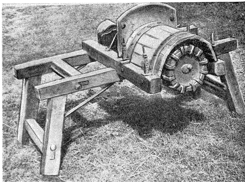
5 pav. Mašina linų galvoms kulti
