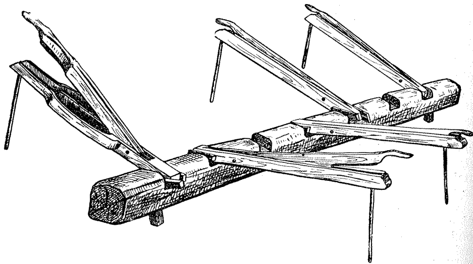
6 pav. «Ožys» ir žemaitiški mintuvai Skuodo raj., Užluobės apyl., Krakų k.
