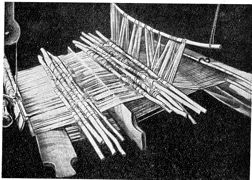
29 pav. Pagalbinių nytelių perskyrimas lentutėmis Dotnuvos raj., Digraičių k.
