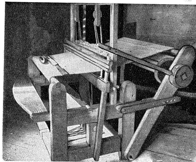
27 pav. Patobulintos sustumiamosios staklės
