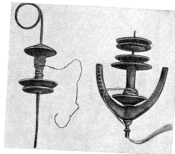
18 pav. Špūlė su špūliauninku ir špūlė, užmauta ant sparno ašies su stricke
