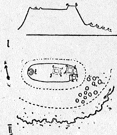
6 pieš. „Džiūgo kalnas.“ Telšių apyl. Skersavaizdis ir planas.
