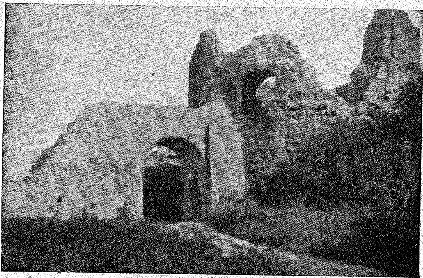
68 pieš. Kauno pilies griuvėsiai.
