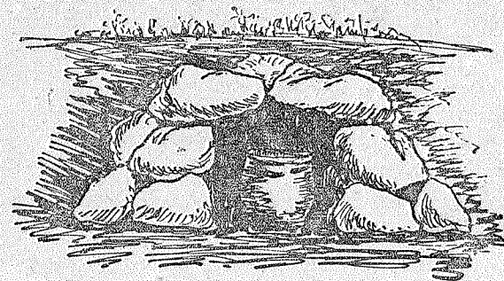
50 pieš. Akmenis laikmečio kapas. Samuliava, Žaslių valsč., Trakų apskr.
