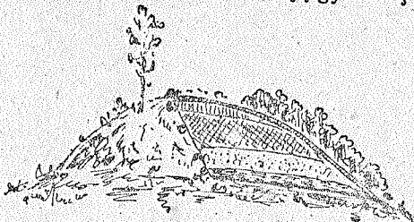
15 pieš. Slizčių piliakalnio, Veprių val., Ukmergės aps., skersavaizdis (e — senas pylimas, d — senas kultūros sluoksnis, c — naujas pylimas, b — naujas kultūros sluoksnis, a — gruntas).
