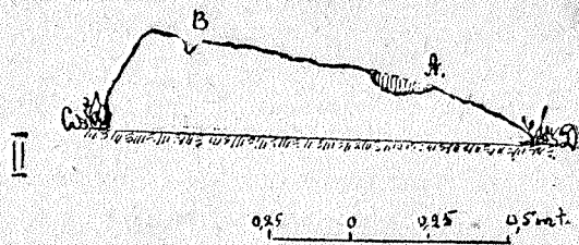
58 pieš. „Kryžiaus“ akmens planas ir skersavaizdis (žūr. 33, 57 pieš.).
