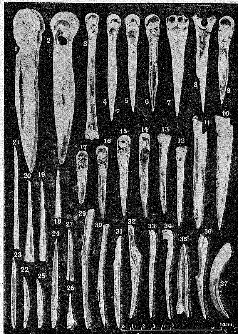
67 pieš. Kaulo padarai iš kultūros sluoksnių Aukštaičių piliakalnių.
