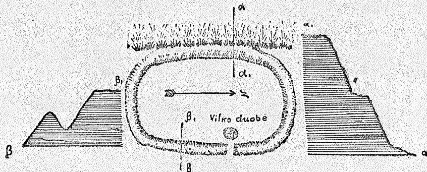
24 pieš. Kupiškio piliakalnio planas ir pūviai
