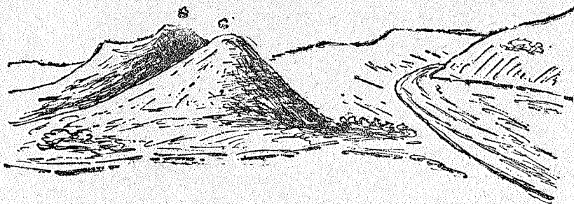
30 pieš. Vienuolyno kalnas, Alytaus apskr.
