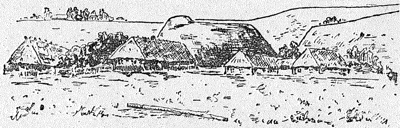
19 pieš. Patarionių piliakalnis, Alytaus aps.
