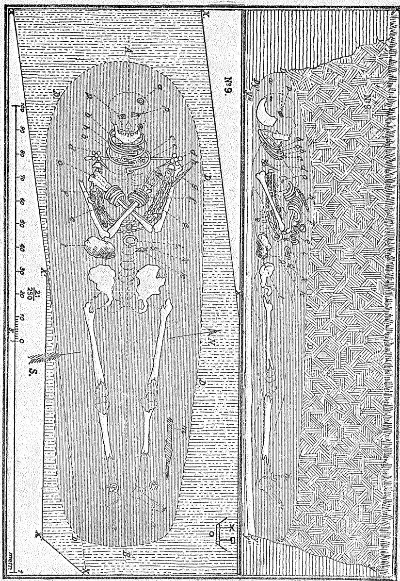
52 pieš. Jasnogurkos senkapio kapa N. 9 skersavaizdis ir planas, Josvainių valsč., Kėdainių apskr.
