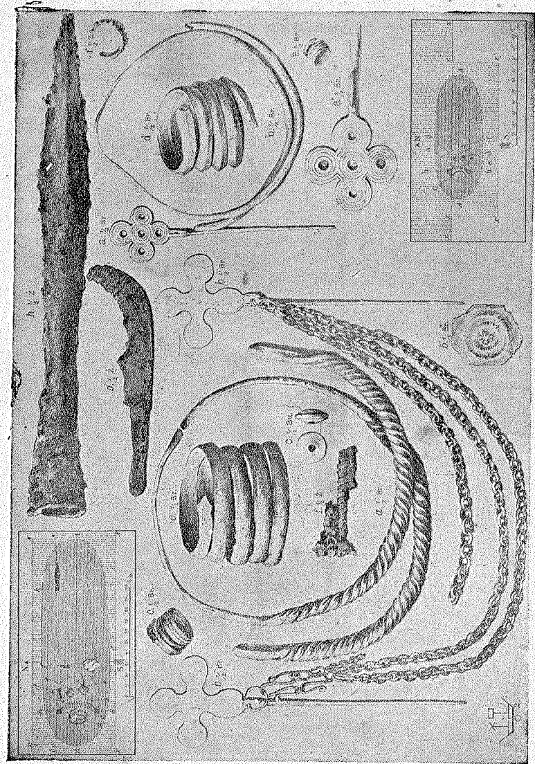
62 pieš. Geležies ir žalvario padarai iš Jasnogurtkos senkapio (žūr. 45 pieš.).
