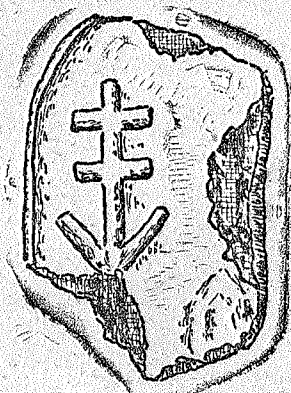
66 pieš. Koklio šukė iš Margio pilies griuvėsių, Pūnioj. Ornamentas, buvęs labai žinomas senovėj, — „Vytties kryžius“.
