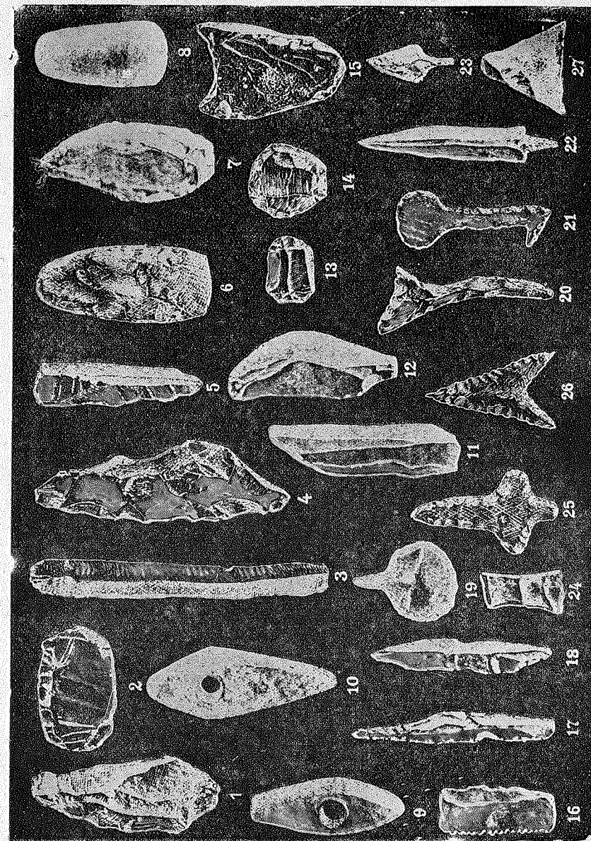
59 pieš. Akmens padarai, tipingi Lietuvos akmens amžiaus kultūrai.
