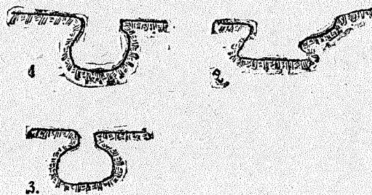
4 pieš. „Kultūros“ rūsių pavyzdžiai; juose gyvendavo akmens laikmetyje.
