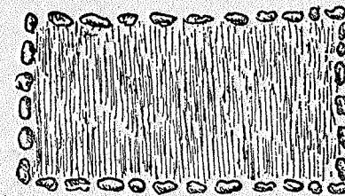
47 pieš. Kaniuckų senkapio kapas. Aluntos valsč., Utenos apskr.
