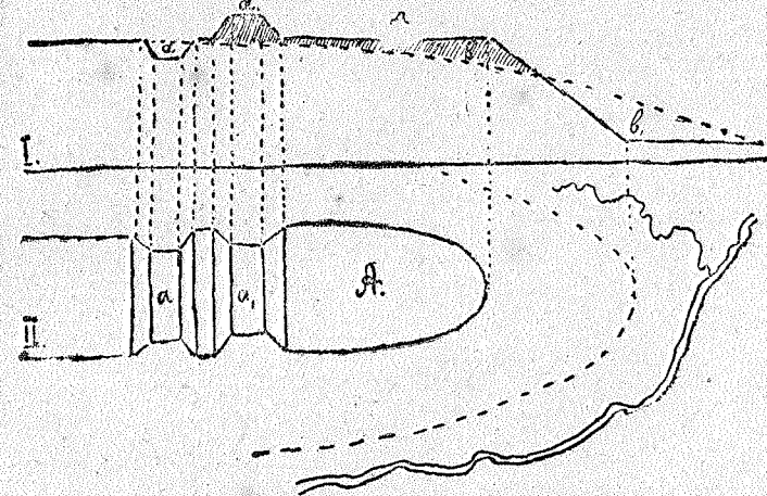
18 pieš. Vėlesnių laikų piliakalnių statybos (planas ir skersavaizdis).
