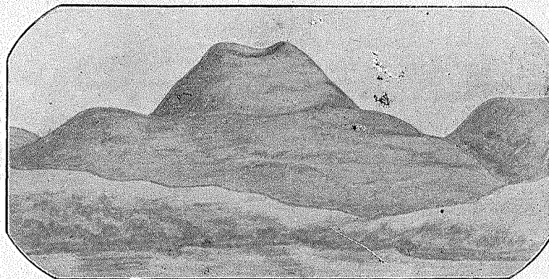
9 pieš. Rumbonių piliakalnis, Kalvarijos aps.
