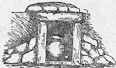
49 pieš. Akmens laikmečio kapas Lenkijoje.
