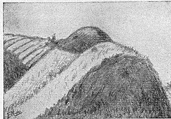
29 pieš. „Žydų kapai“, tikišinių apeigų piliakalniai prie Papatų pilies, Žaslų valsč., Trakų apskr.
