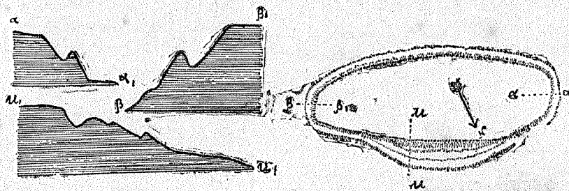
26 pieš. Girždutos piliakalnio planas ir pylimų pūtviai.
