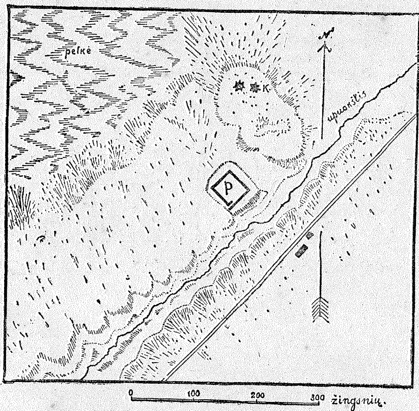
23 pieš. N. Varionų piliakalnio apylinkės schema (Švenčionių aps.).
