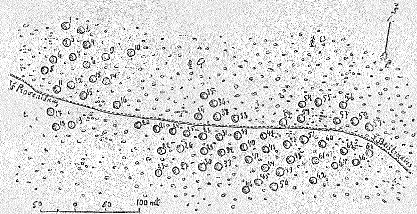
45 pieš. Guronų kapyno schema, Kauno apskr., Rumšiškų valsč.
