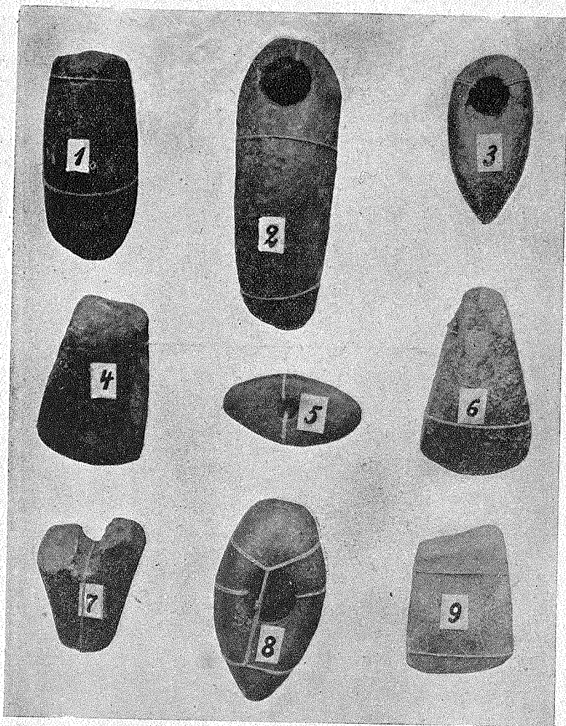
60 pieš. Kirveliai ir plaktukai, tipingi Lietuvos akmens kultūros laikmečiui.
