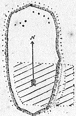
28 pieš. Pilenų piliakalnio planas (Kėdainių apylinkės).
