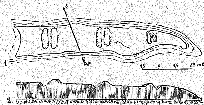
10 pieš. Račkiškių piliakalnio planas ir skersavaizdis. Atriogalos apyl.
