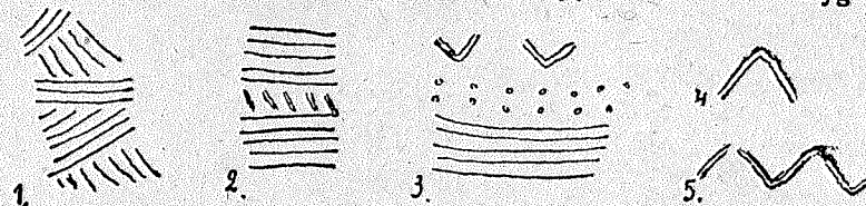
64 pieš. Lietuvos varlo kultūros laikmečio molinių puodų ornamentai.
