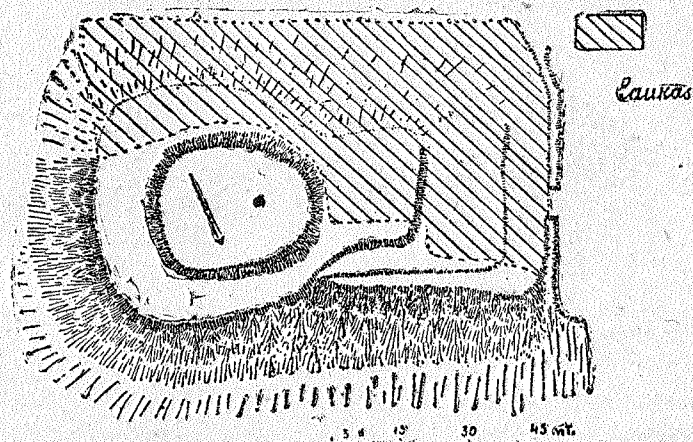
22 pieš. Bilonių piliakalnio planas.
