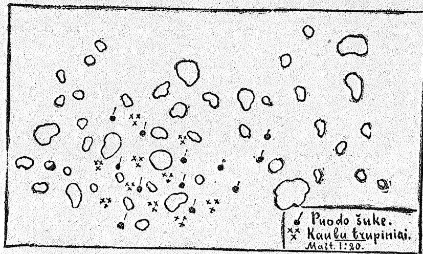
5 pieš. Akmens kultūros laikmečio kapo akmenų planas. Rūšių sėdyba.
