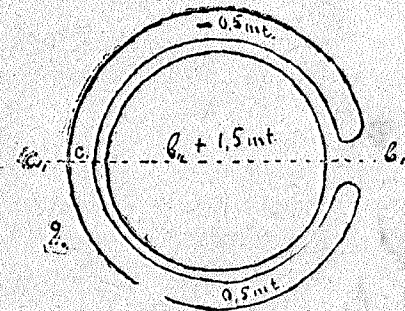
42 pieš. Guronų kapyno kurgano N. 17 skersavaizdis ir planas.
