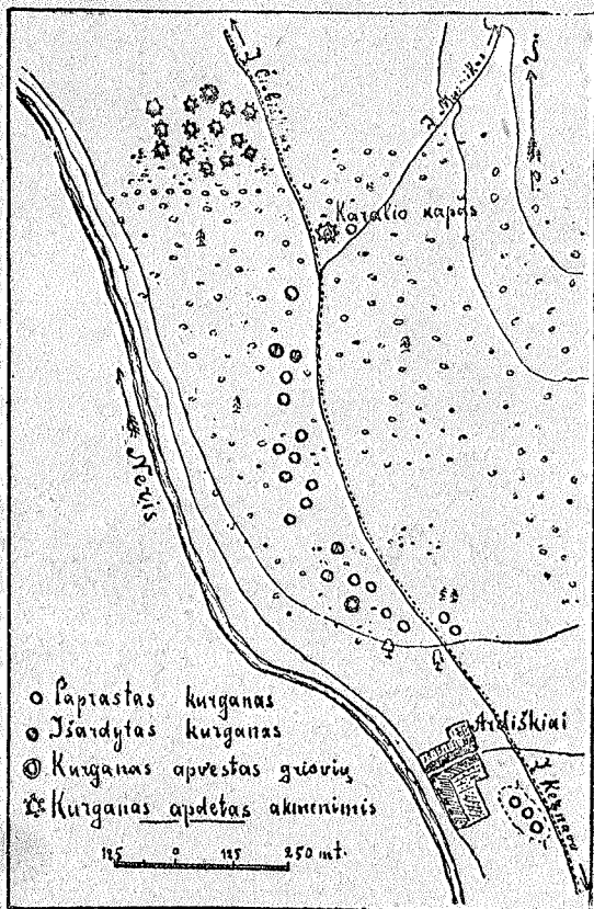
46 pieš. Ardiškų kapyno schema, Kernavos apylinkėj.
