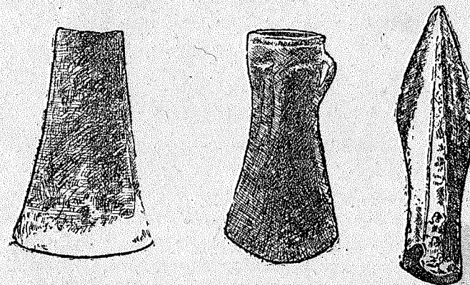
61 pieš. Žalvario padarai, tipingi Lietuvos žalvario kultūros laikmečiui, atrasti Merkio ir Nemuno upių srityse.
