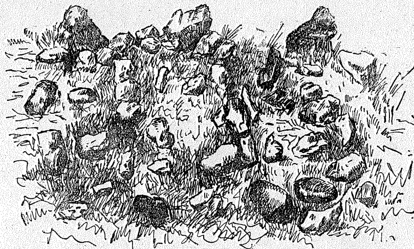
48 pieš. Vilniaus gub. senkapis.
