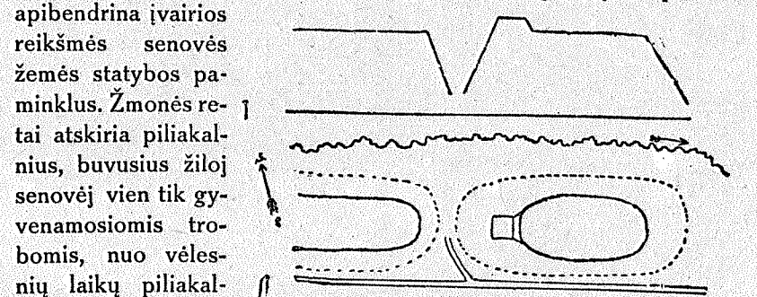
7 pieš. Veliunos pilis. Skersavaizdis ir planas.
