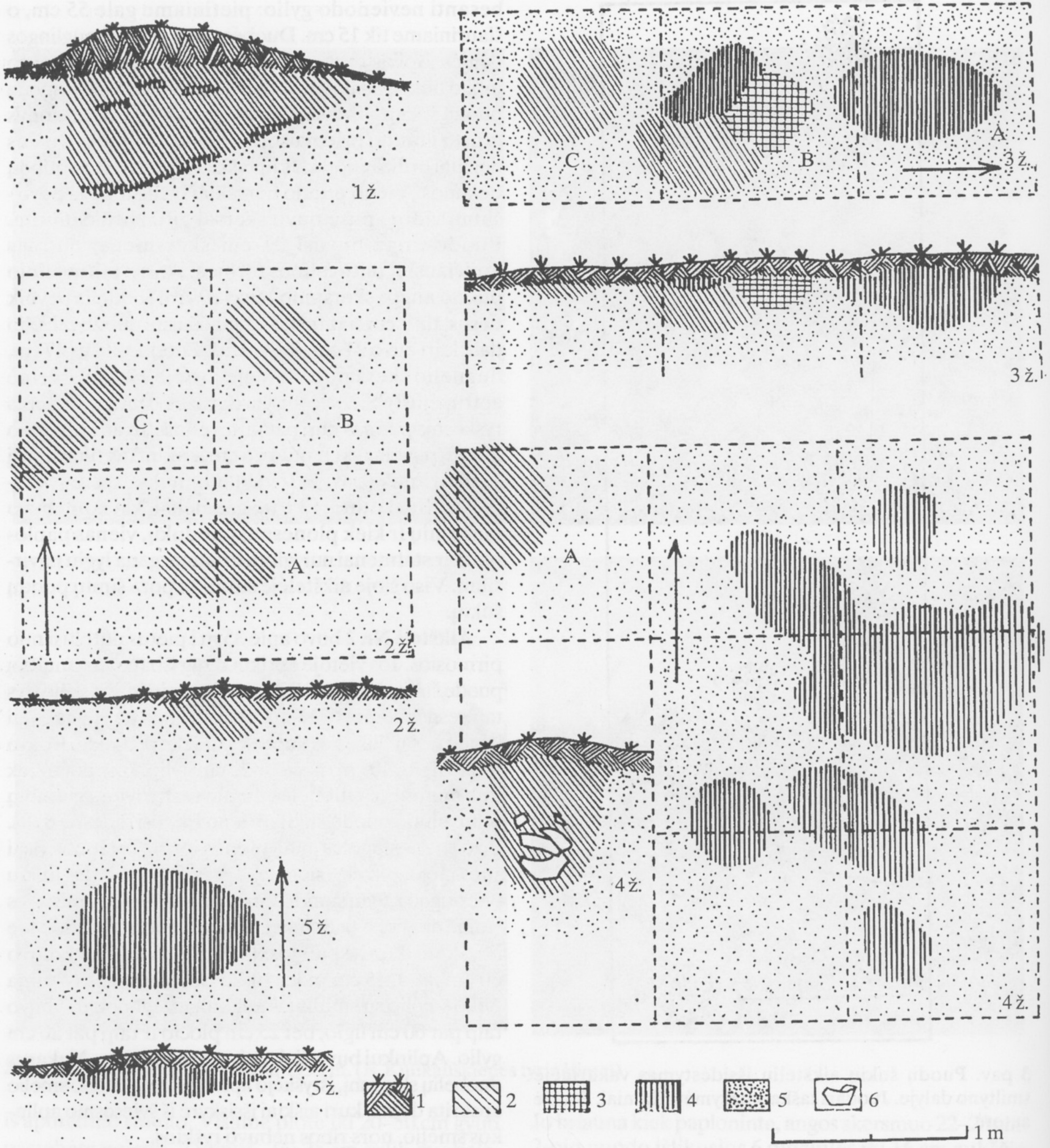
4 pav. Puodų šukių aikštelių Nr.1-5 planai: 1 – velėna, 2 – šviesiai pilkas smėlis, 3 – tamsiai pilkas smėlis, 4 – degėsiai ir suodžiai, 5 – baltas smėlis. Braižė autorė
