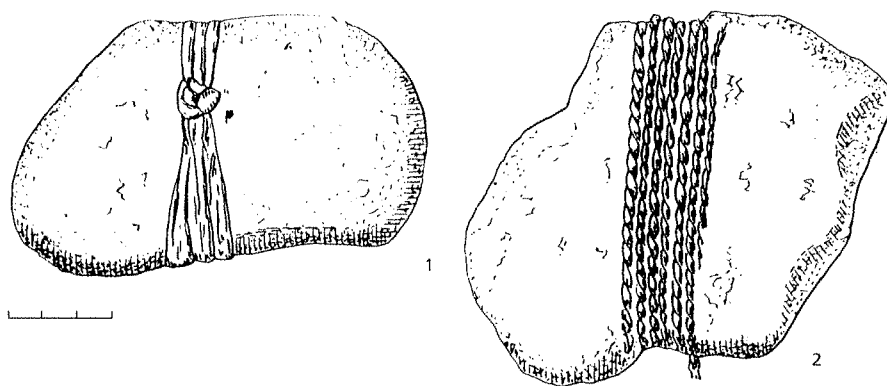
215 pav. Šventosios 3-iosios rad. tinklų pasvarelėliai, perrišti liepos karna ir karnos virvelėmis (LNM)
