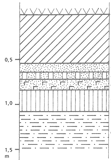
226 pav. Šventosios 5-osios rad. 6-ojo šurfo pjūvis. 1 – durpės, 2 – smėlis, 3 – smėlis su gijija – kultūrinis sluoksnis, 4 – geležingas smėlis, 5 – gijija, 6 – aleuritai su smėliu
