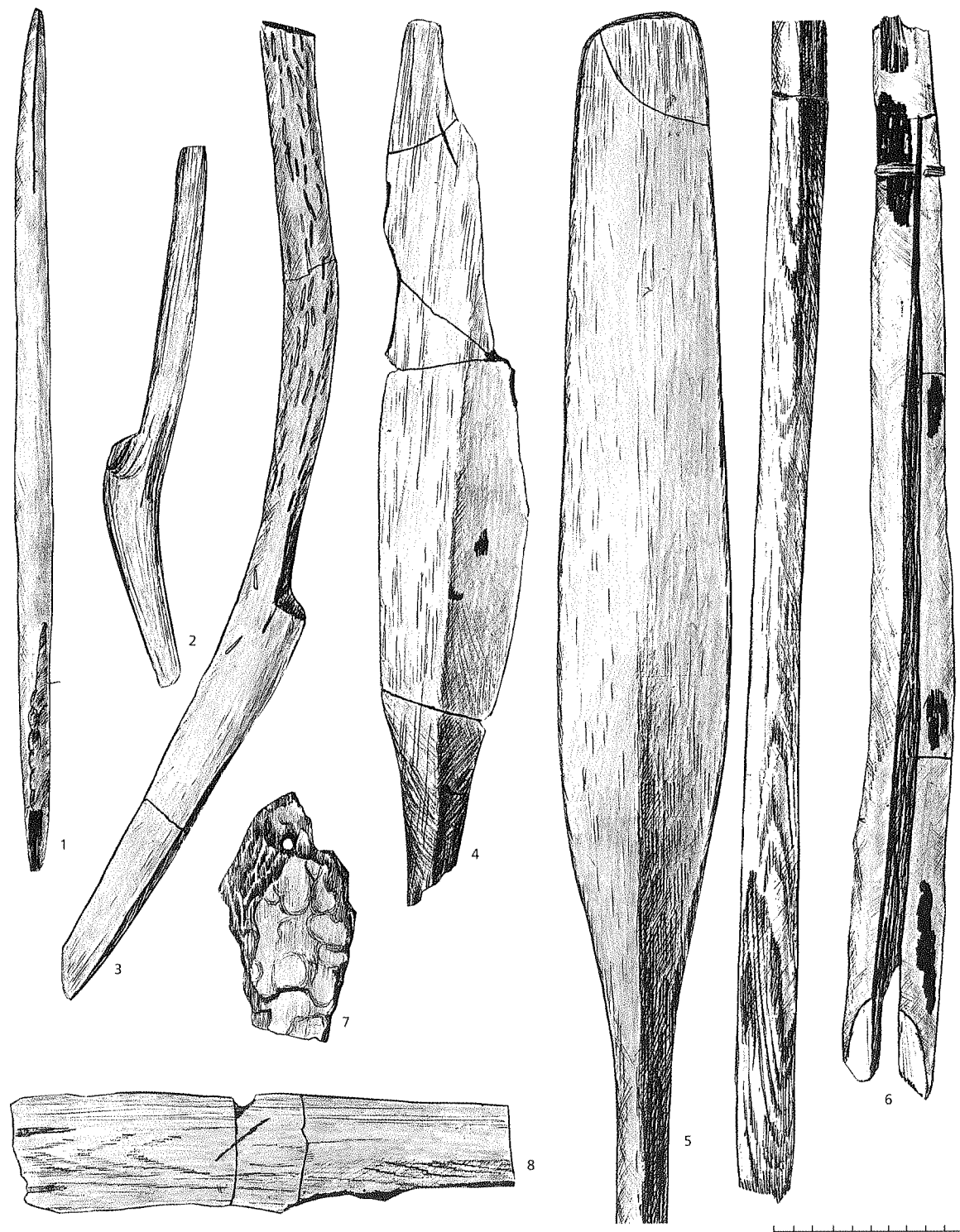
222 pav. Šventosios 3-iosios rad. medžioklės ir žūklės medinės priemonės. 1 – kv. 6r, 2 – kv. 13l, 3 – kv. 12l, 4 – kv. 13l, 5 – kv. 5n, 6 – kv. 12l, 7 – kv. 5n, 8 – kv. 12l (LNM)
