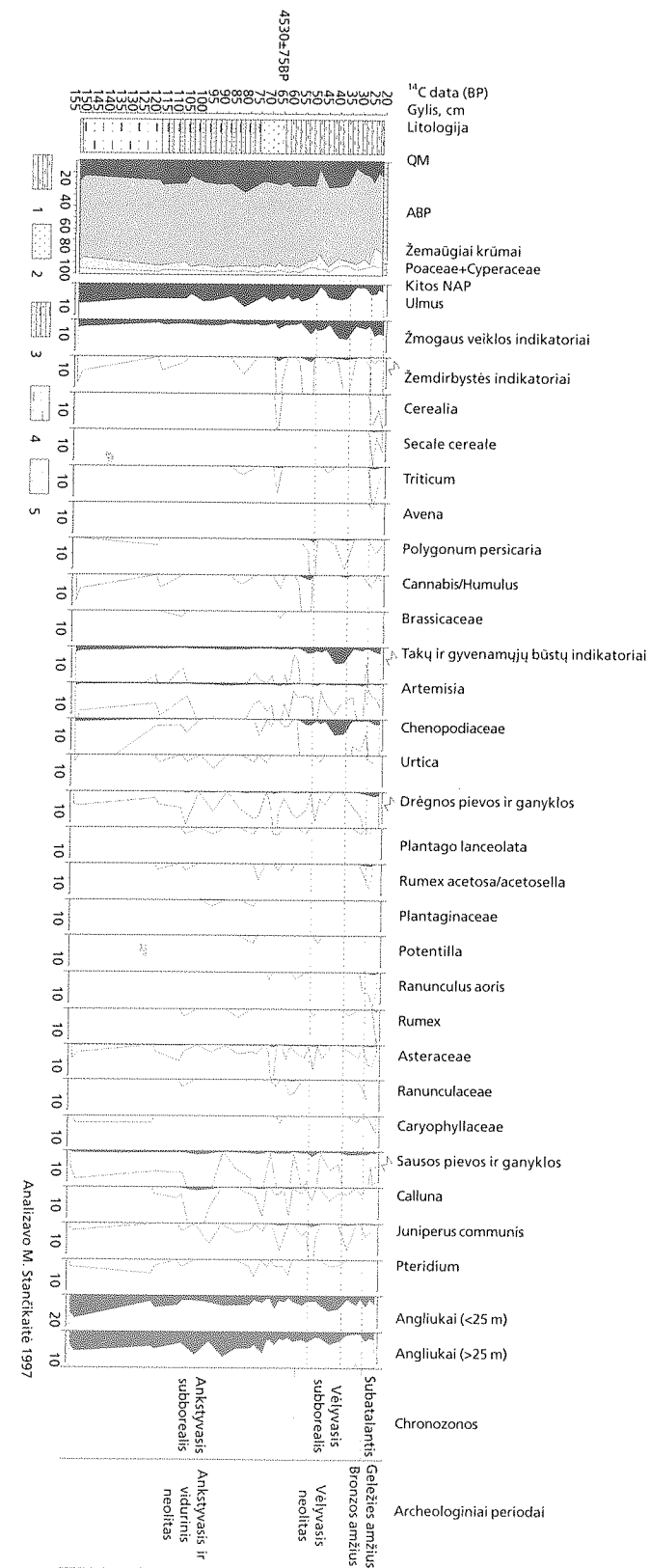
235 pav. Šventosios 6-osios rad. žiedadulkių-sporų analizė, atspindinti gyventojų poveikį aplinkai. 1 – aleuritinga gitija, 2 – smulkus smėlis, 3 – smulkus aleuritingas smėlis, 4 – aleuritingas smėlis, 5 – vidutinis smėlis (analizavo M. Stančikaitė)
