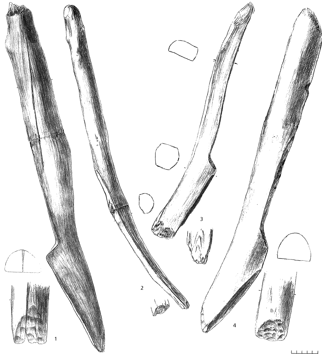
289 pav. Šventosios 6-osios rad. mediniai rankiniai arklai. 1 – kv. 51g–h, 2 – kv. 48j, 3 – kv. 46i, 4 – kv. 16h (LNM)
