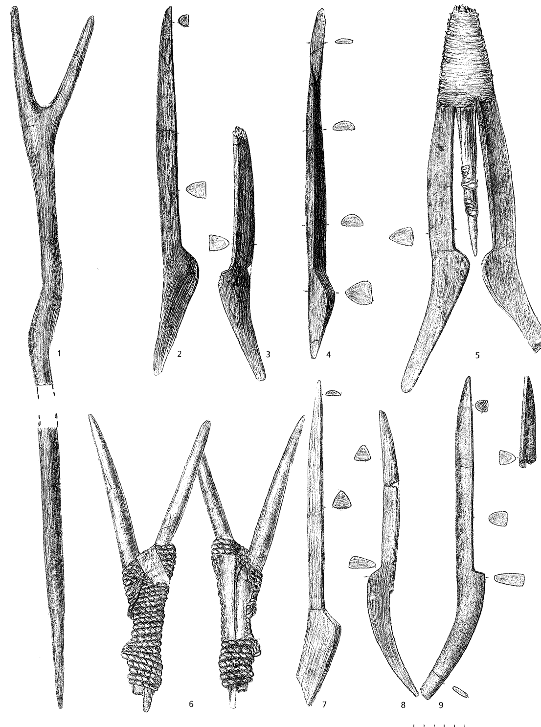
186 pav. Šventosios 4B rad. šakės žuvims gaudyti. 1 – kv. 4/62v, 2 – kv. 4/44v, 3 – kv. 4/44z, 4 – kv. 4/53u, 5 – kv. 4/34u, 6 – kv. 4/37z, 7 – kv. 4/64z, 8 – kv. 4/63z, 9, 10 – kv. 4/13p (LNM)
