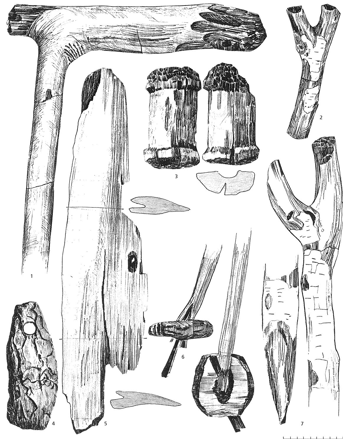
181 pav. Šventosios 2/4B mediniai dirbiniai: kūle (1), dvišakiai (2, 7), kirvio mova (3), plūdė (4), luoto (?) dalis (5), atspiriamoji lazda (6). 1 – kv. 2x/8c, 2 – kv. 2x/12d, 3 – kv. 2z/10a, 4 – kv. 2x/3b, 5 – kv. 2x/1b, 6 – kv. 2y/13b, 7 – kv. 2y/15–16b (LNM)
