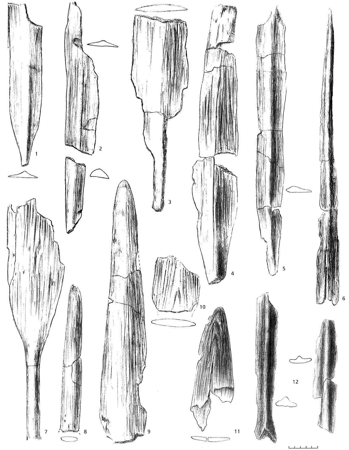
285 pav. Šventosios 6-osios rad. irklai. 1 – kv. 27f, 2 – kv. 38j, 3 – kv. 28f, 4 – kv. 29i, 5 – kv. 52i, 6 – kv. 49j, 7 – kv. 28k, 8 – kv. 26g, 9 – kv. 30e, 10 – kv. 27f, 11 – kv. 55i, 12 – kv. 74i (LNM)
