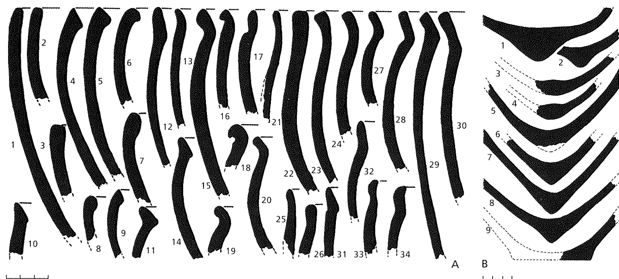
207 pav. Šventosios 3-iosios rad. puodų kaklelių (A) ir dugnelių (B) pjūviai
