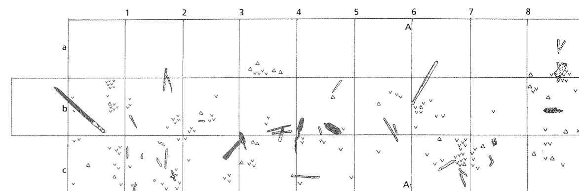
132 pav. Šventosios 2-osios rad. y perkasos planas ir pjūvis. 1 – smėlis, 2 – durpės, 3 – gitijos luobo sluoksnis, 4 – detritinė gitija – kultūrinis sluoksnis, 5 – gulinčios kartys, 6 – mediniai dirbiniai, 7 – puodų šukės, 8 – tinklų pasvarėliai
