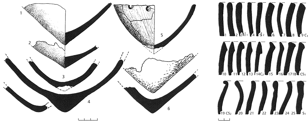
158 pav. Šventosios 2/4B rad. puodų kaklelių ir dugnelių pjūviai
