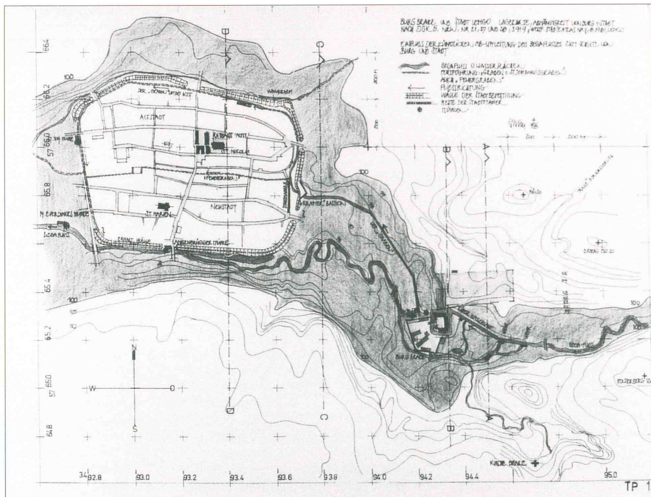
Abb. 4. Lageplan der Stadt Lemgo und der Burg Brake und ihrer Abhängigkeiten. Die Umleitung der natürlichen Wasserläufe zum Schutz und zur Versorgung der Stadt sind dargestellt. Die grau angelegte Fläche markiert die Höhenebene 100,00m NN. Gemeinsame Gründung durch Bernhard zur Lippe um 1190
