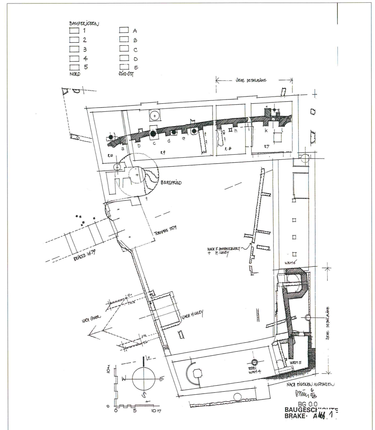
Abb. 1. Grabungsplan Burg/Schloss Brake 1998. Dargestellt sind die Mauerfunde der mittelalterlichen Burganlage, entstanden in der Ausbauphase Bernhards II. unter dem heutigen Renaissanceschloss
