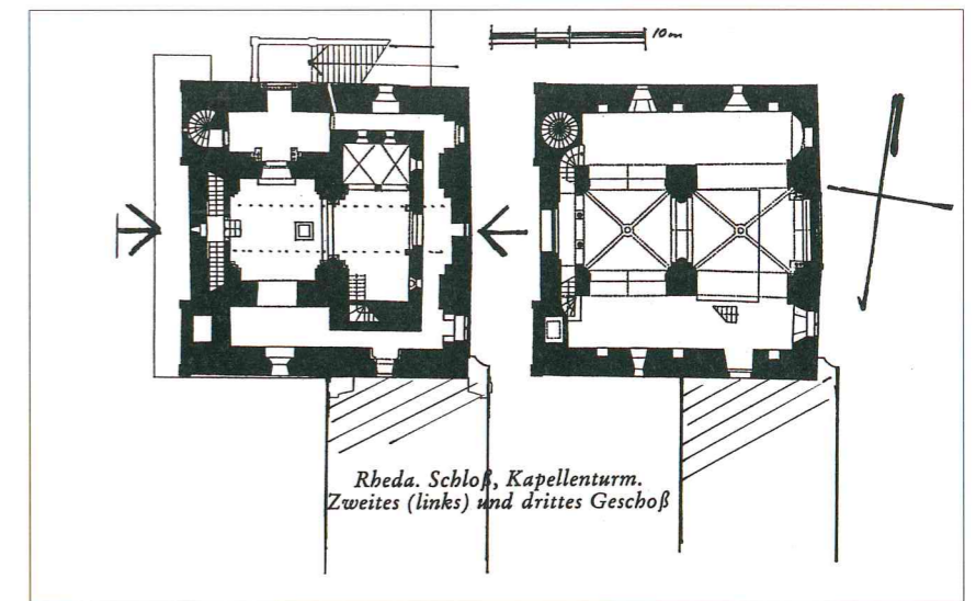
Abb. 6. Tortum Rheda. Deutschland, Nordrhein-Westfalen. Um 1220 Bernhard II., (oder Hermann II.) zur Lippe. Grundriss 2. und 3. Geschöß
