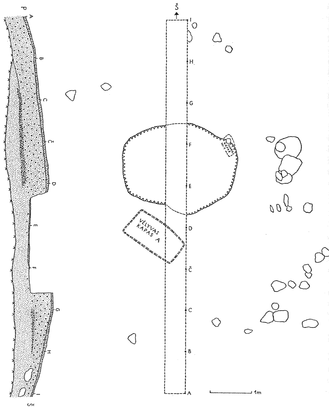
80 pav. V pilkapis planas Abb. 80. Plan des Grabhügels V.
