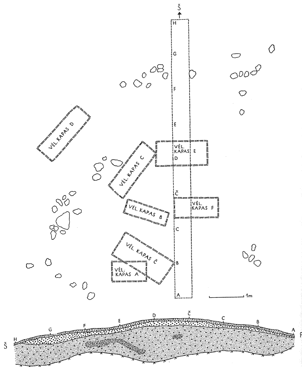
87 pav. XIX pilkapio planas Abb. 87. Plan des Grabbügels XIX.
