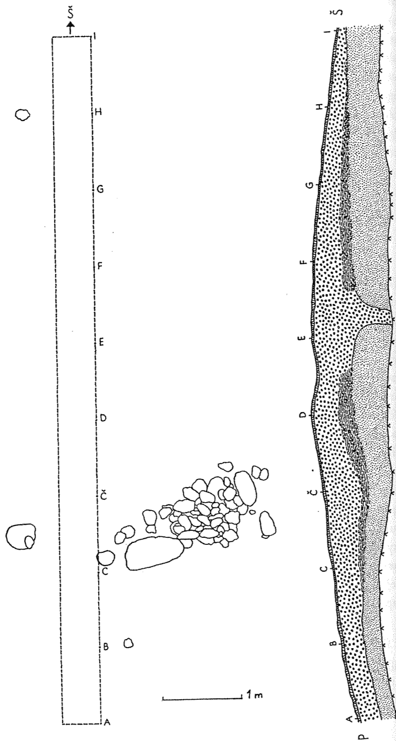
76 pav. I pilkapio planas Abb. 76. Plan des Grabbügels I.
