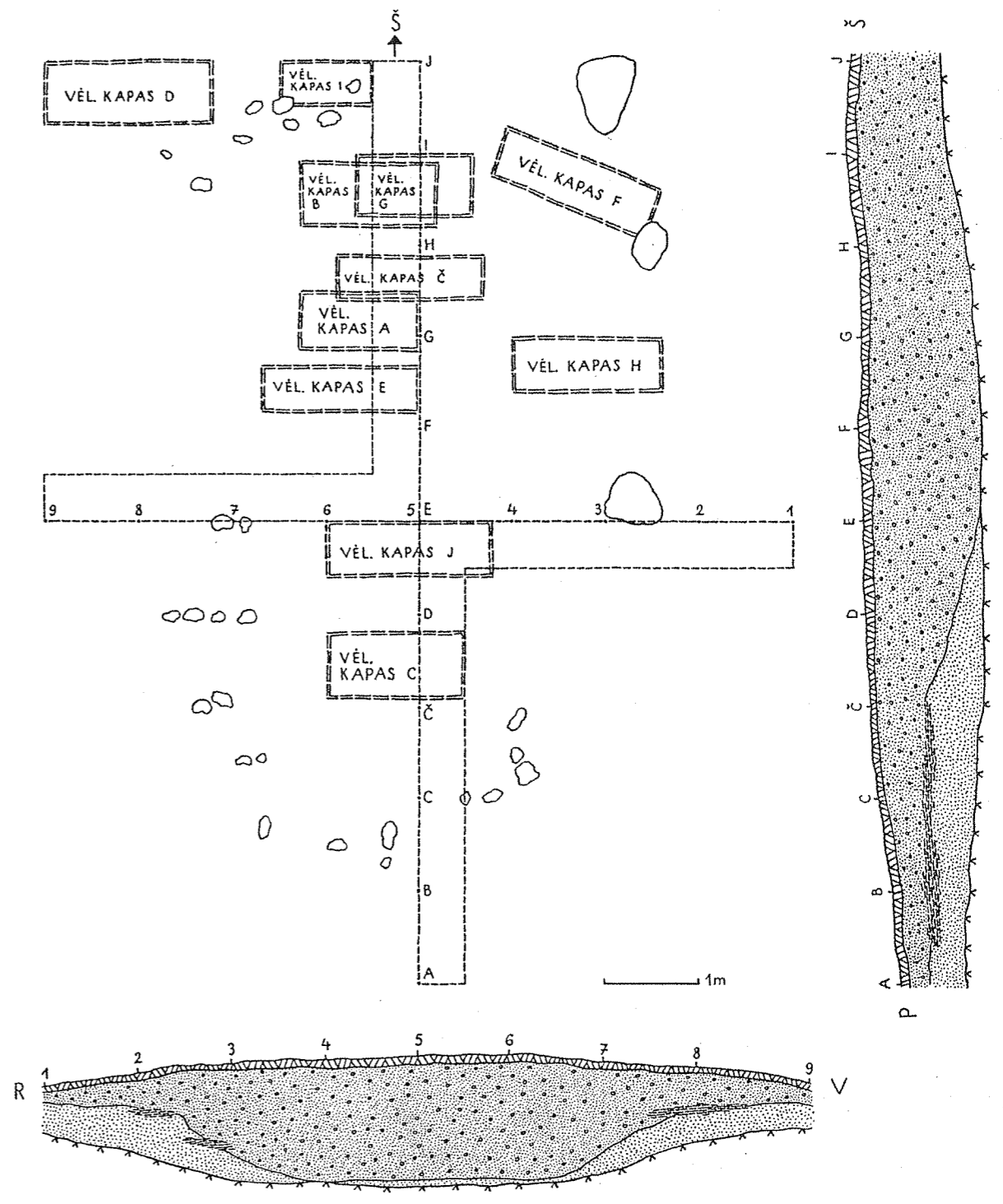
84 pav. XV pilkapio planas Abb. 84. Plan des Grabhügels XV.
