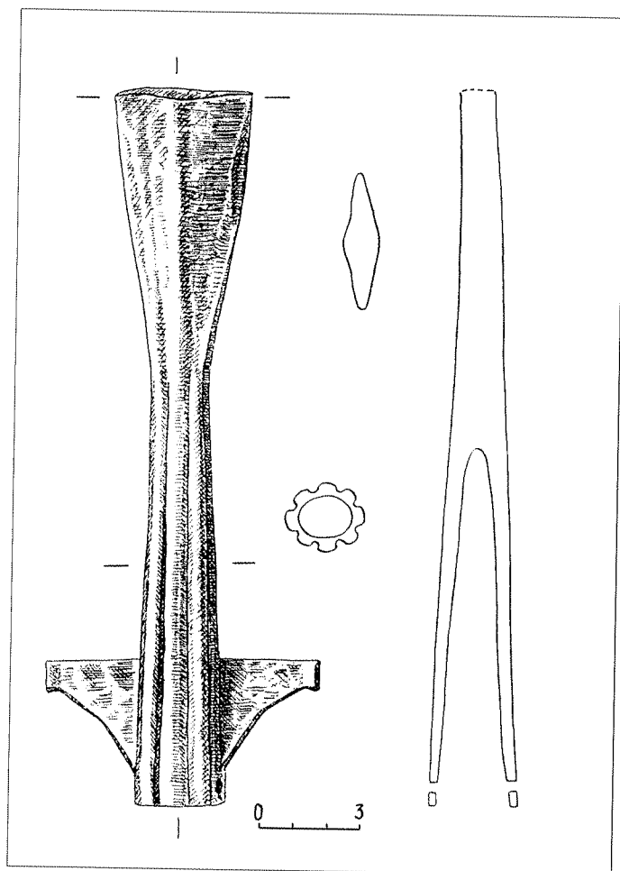
62 pav. Karių elito ginklas – ietigalis su sparneliais (Marvelė, ats. radinys)
