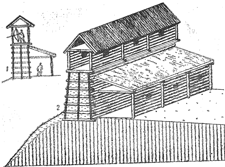
13 pav. Rekonstruotas Vilniaus Kreivosios pilies II tūkstantmečio pačios pradžios (XI—XIII a.?) gynybinis įrenginys (rekonstravo autorius ir architektas S. Lasavickas): 1 — įrenginio skersinis pjūvis, 2 — vaizdas iš šono
