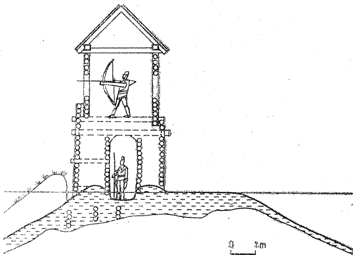
15 pav. Rekonstruota 1390 m. sudegintos Vilniaus Kreivosios pilies gynybinė siena (rekonstravo autorius ir architektas S. Lasavickas)
