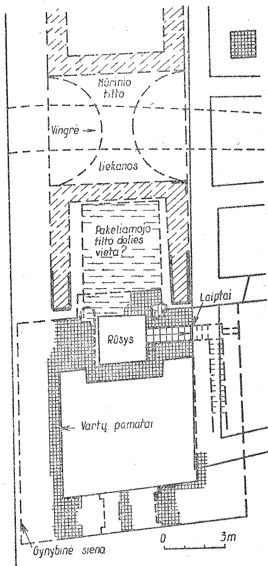
10 pav. „Vilniaus“ vartų tyrinėtos dalies planas (braižė architektas S. Lasavickas)
