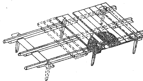
3 pav. Rekonstruotas medinis kelio grindinys Senojo arsenalo teritorijoje (architektas S. Lasavickas)
