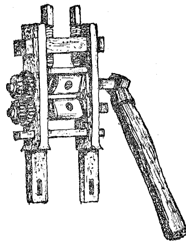
25 pav. Valcavimo staklės su keičiamais štampais, pritaikytos monetoms gaminti
