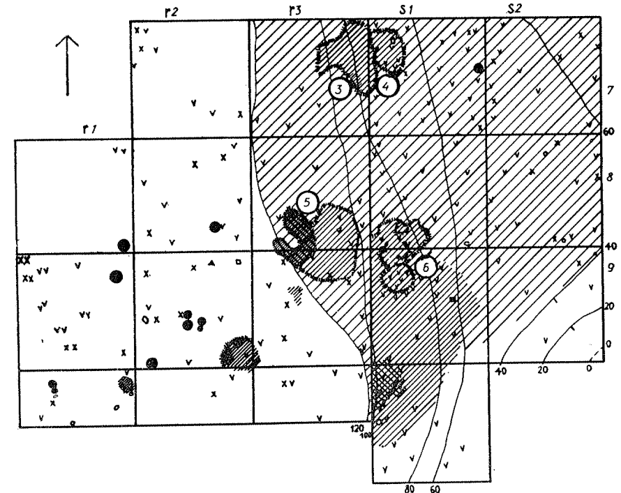
6. 2-os iškarpos planas
