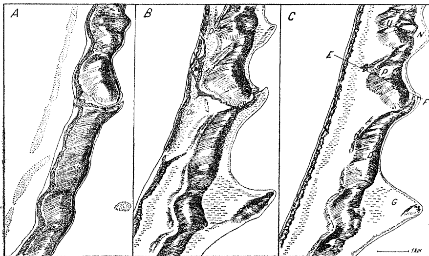
19. A. Nidos sąsiauris per paskutinę Litorinos jūros transgresiją (apie 2700 m. pr. m. e.) B. Sąsiauris per Limnės jūros regresiją (apie 2200 m. pr. m. e.): L — lagūna, S — sąsiauris, Dr — sezoniški druskingi ežerėliai (pagal R. Kunska) C. Parnidžio kopos apylinkės dabar: D — Didžioji (Ilgoji, Sklandytojų) kopa, P — Parnidžio kopa, U — Urbo kopa, G — Grobšto ragas, N — Nidos gyvenvietė, E—F — skersinis nerijos profilis
