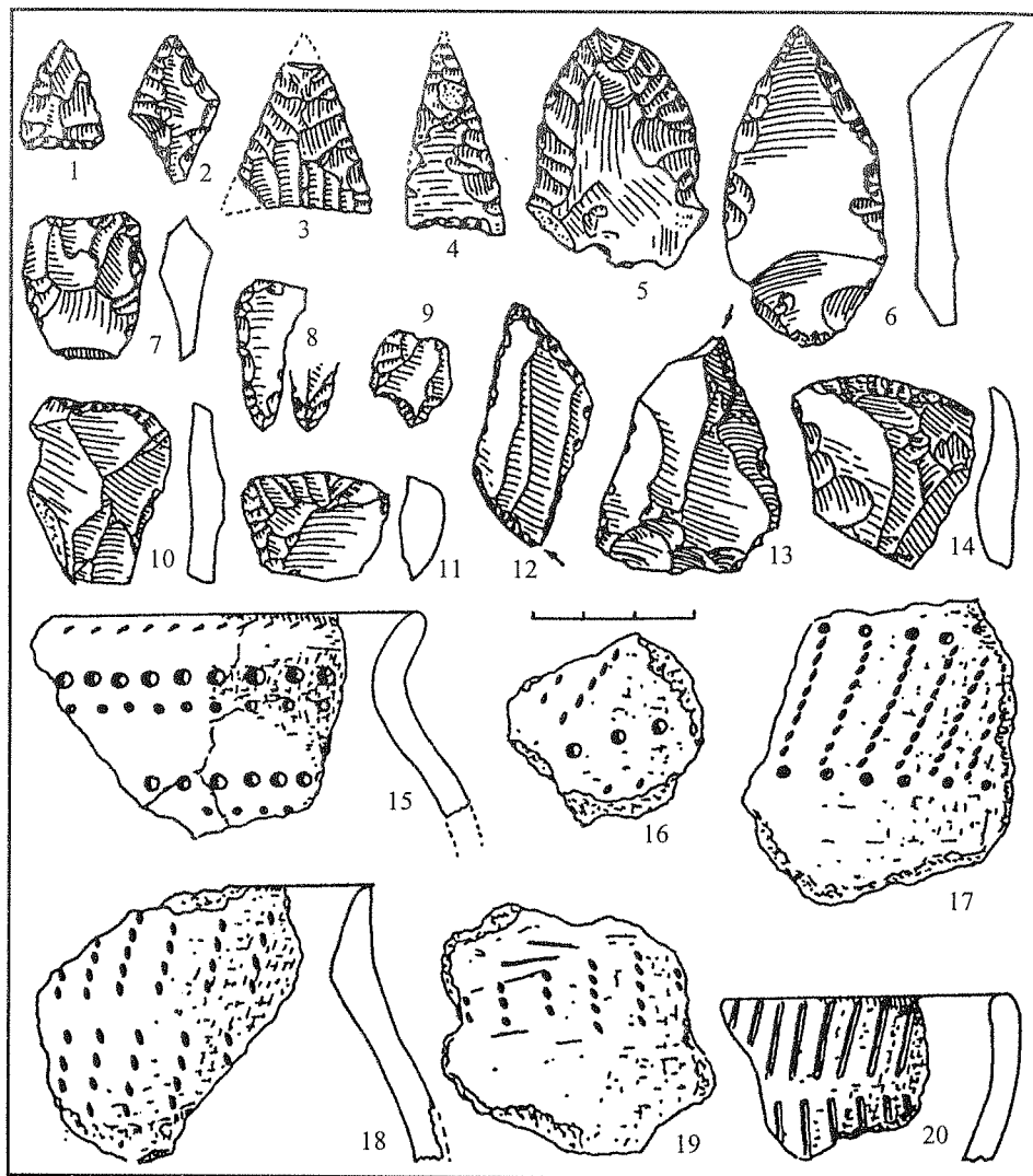
141 pav. Pagrindiniai Šventosios 26-osios gyv. radiniai: 1–4 – strėlių antgaliai, 5, 6 – peiliai, 7 – kaltelio ašmenėlis, 8, 9 – gražteliai, 10, 11, 14 – gremžtukai, 12, 13 – rėžtukai, 15–20 – keramika (LNM)
