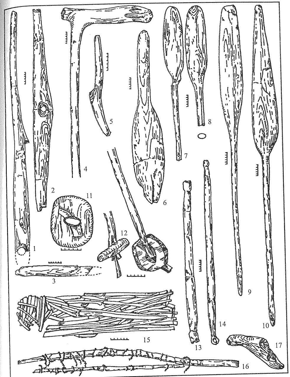
93 pav. Šventosios gyvenviečių mediniai žūklės įrankiai: 1, 2 – butiniai, 3 – butinius jungiantis skersinis, 4 – kūlė, 5 – šakių žuvims gaudyti dalis, 6–10 – irklai, 11, 12 – lazdos su skridiniais, 13, 14 – branktai, 15, 16 – bučių dalys, 17 – samtelis (1–3, 6, 14 – 1B gyv., 4, 7, 8, 10–12, 15, 16 – 2B gyv., 5, 9 – 3B gyv., 13, 17 – 23-ioji gyv.) (LNM)
