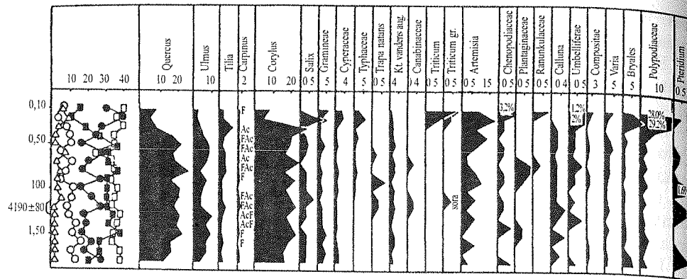
101 pav. Šventosios 23-iosios gyv. žiedadulkių diagrama (N. Savukynienė)
