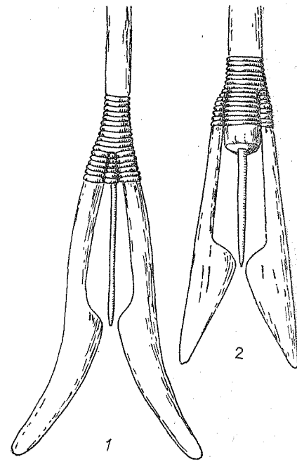
76 pav. Pagal Šventosios 23-os ir 3B gyv. radinius rekonstruotos šakės žuvisms gaudyti
