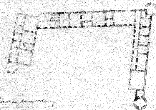
Panemunės pilies šiaurinis fasadas ir pilies planas (iš 1827 m. „Vilniaus gubernijos pilies atlaso“)
