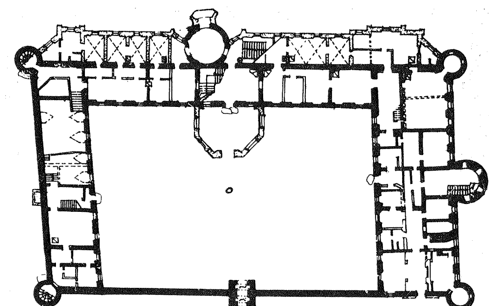
35 pav. Raudonės pilies plano raida
